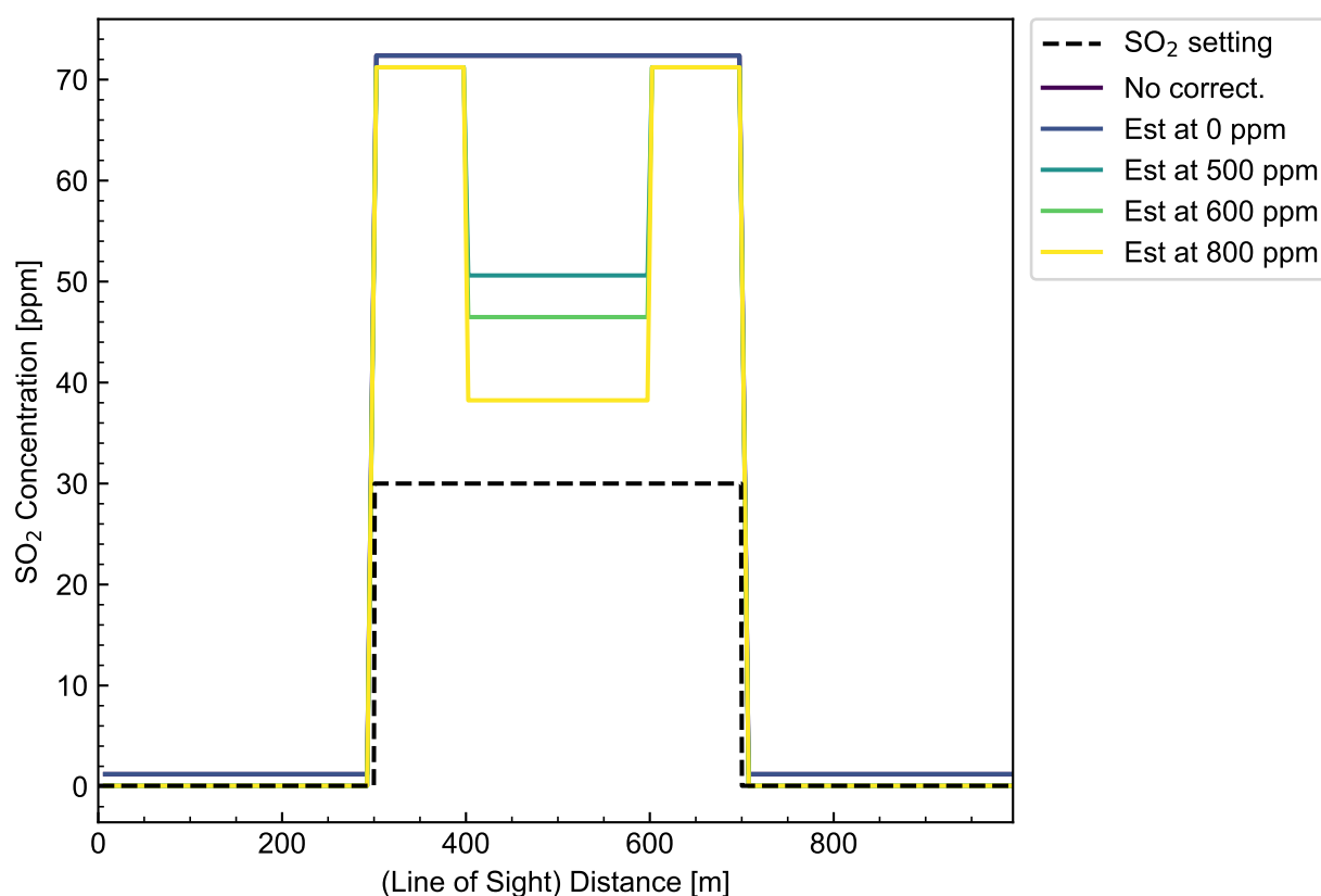
図 3.5: 高濃度区間の一部について H 2 S 補正を行ったラマン DIAL による SO 2 測定シミュレーション
