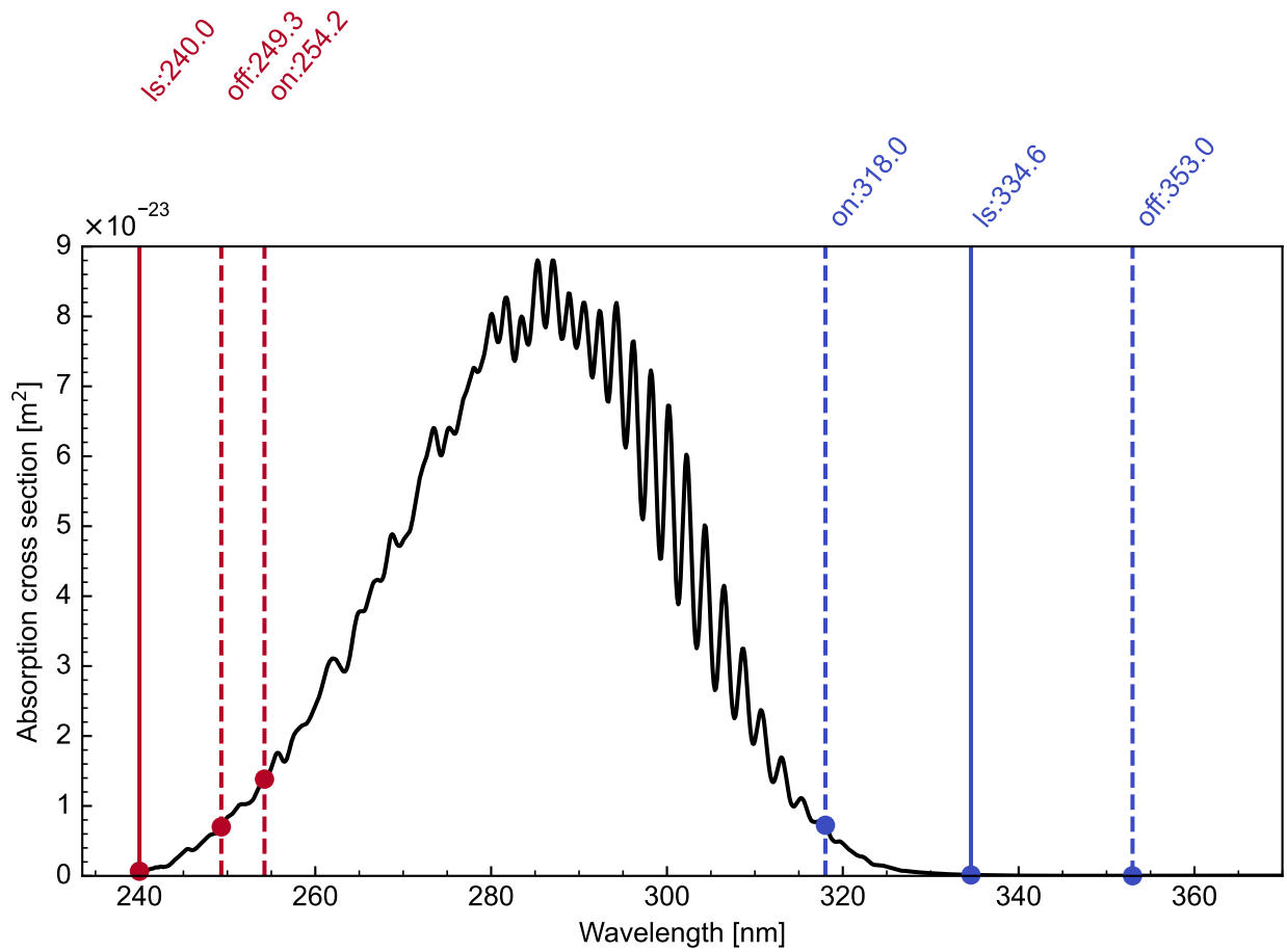
図 2.5: 二つの受信波長構成 ( \text{N}_2 ストークス散乱波長と \text{O}_2 ストークス散乱波長, \text{O}_2 ストークス散乱波長と \text{O}_2 アンチストークス散乱波長) における \text{SO}_2 吸収断面積
