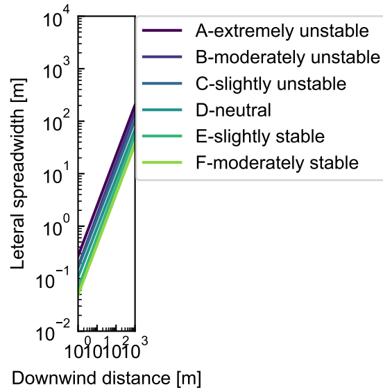
図 4.1: Pasquill-Gifford による水平方向拡散幅 \omega_y の距離特性
