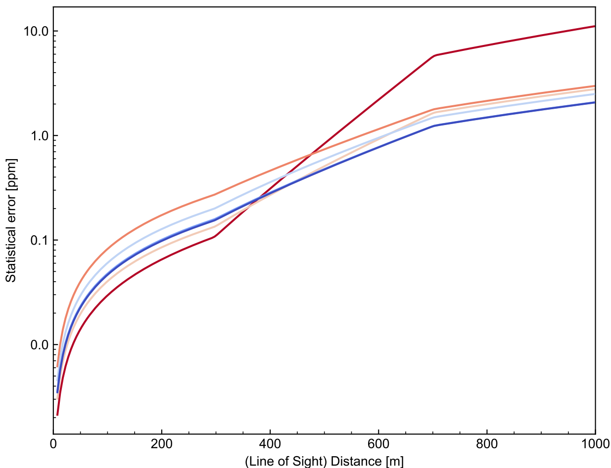
図 2.4: 受信波長の構成による統計誤差の比較
