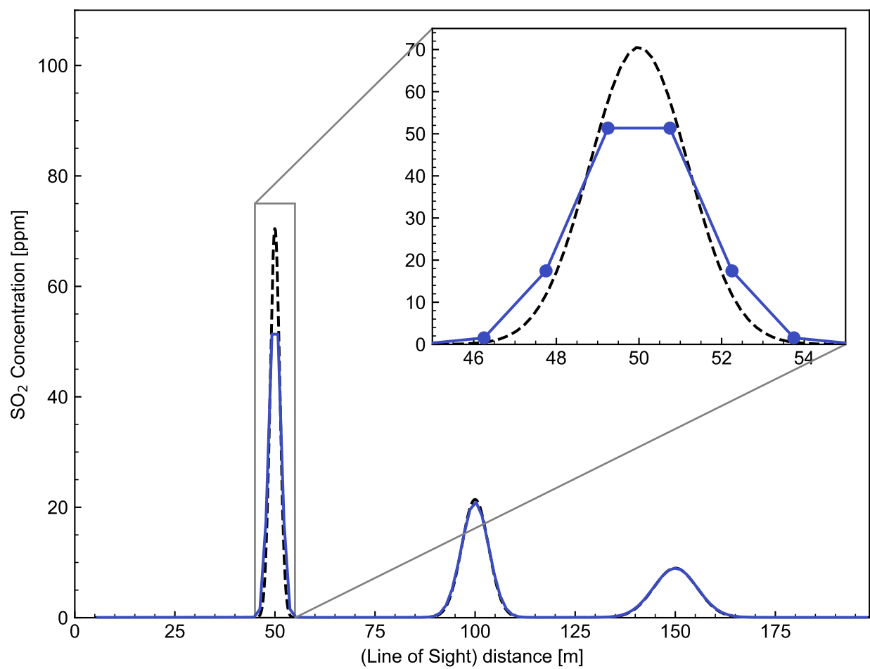
図 4.9: 弱拡散大気条件場における SO 2 測定シミュレーション
