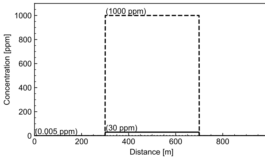
図 3.4: \text{H}_2\text{S} が高濃度の火山ガス分布設定
