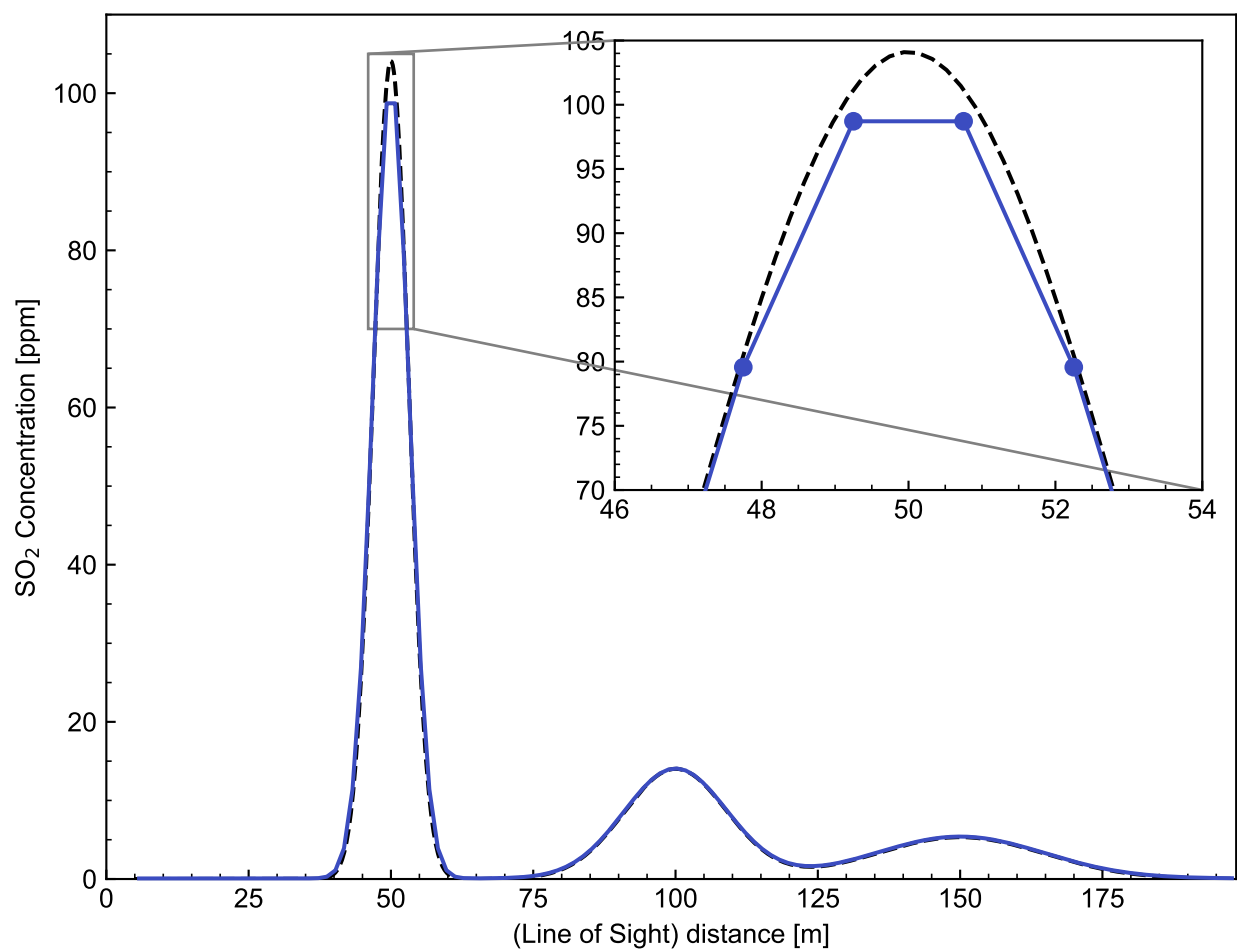
図 4.8: 強拡散大気条件場における SO 2 測定シミュレーション
