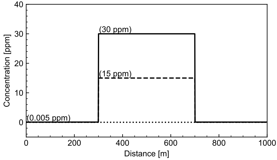
図 2.3: 火山ガス濃度分布の設定
