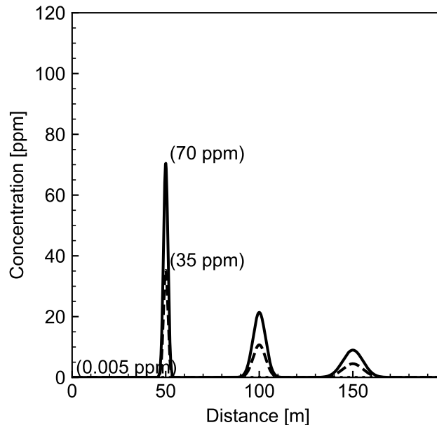
図 4.7: 弱拡散大気条件下における火山ガス濃度視線距離分布
