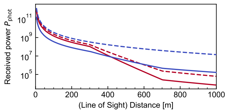
図 2.6: 二つの受信波長構成 ( \text{N}_2 ストークス散乱波長と \text{O}_2 ストークス散乱波長, \text{O}_2 ストークス散乱波長と \text{O}_2 アンチストークス) における受信光子数の距離特性
