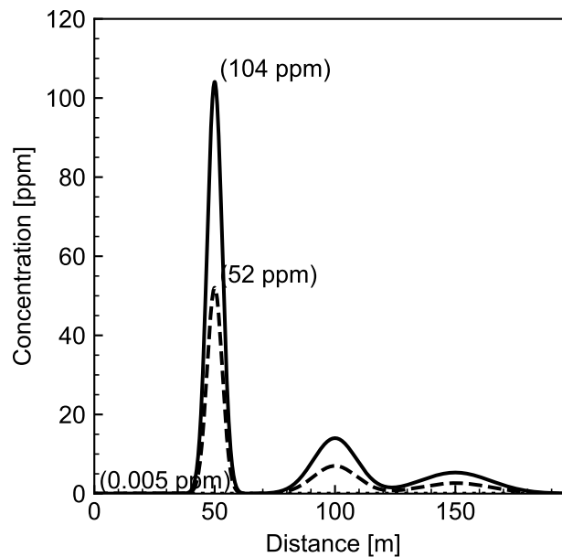
図 4.6: 強拡散大気条件下における火山ガス濃度視線距離分布
