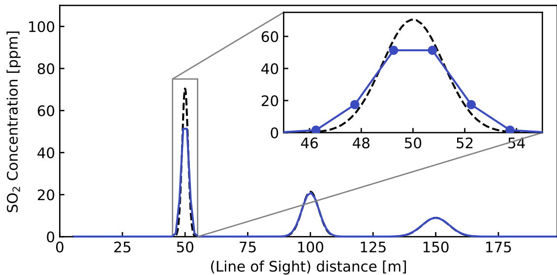
図 4.6: 弱拡散大気条件場における SO 2 測定シミュレーション
