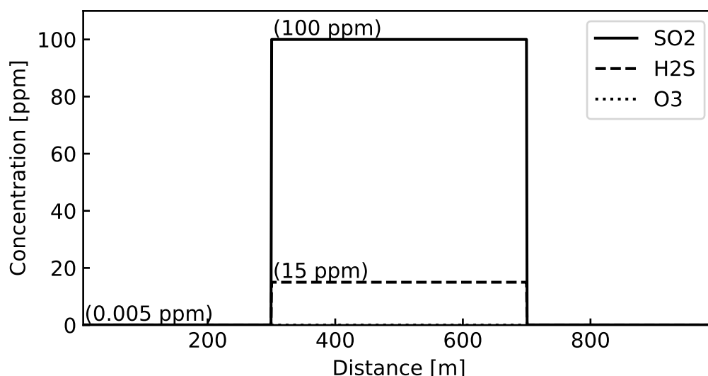
図 3.1: \text{SO}_2 が豊富な火山環境を想定した濃度分布設定
