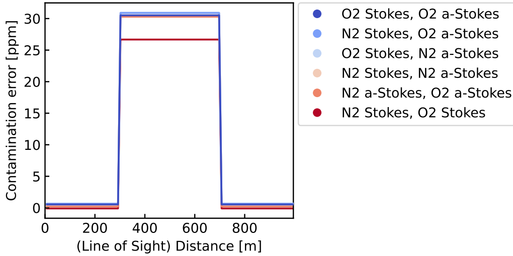
図 2.7: 受信波長の構成による干渉誤差の比較
