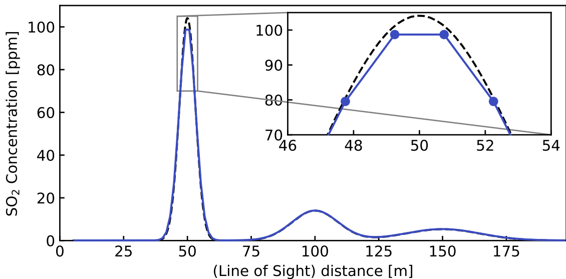
図 4.5: 強拡散大気条件場における \text{SO}_2 測定シミュレーション
