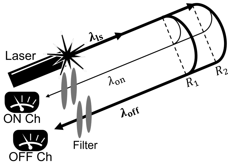
図 5.1: ラマン DIAL の受信側の構成
