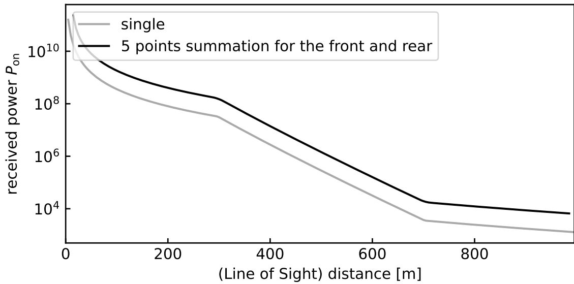
図 3.3: 信号加算前後の受信信号強度の変化
