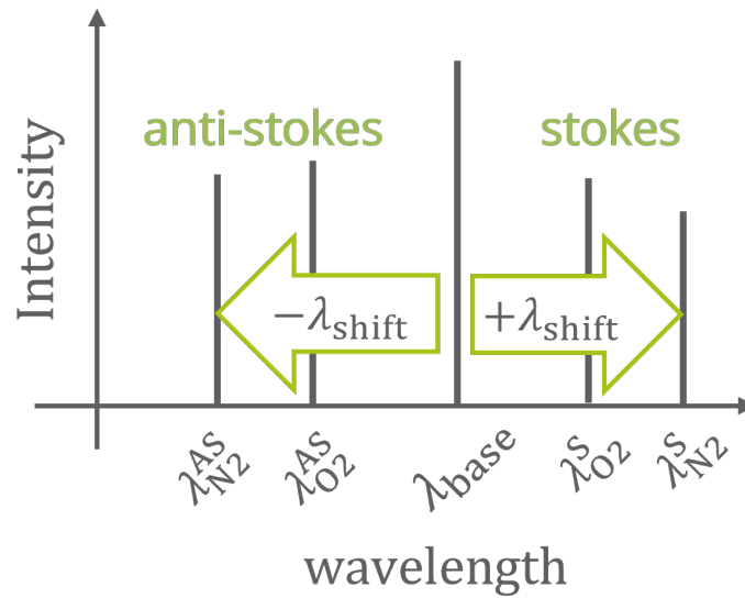
図 2.2: レーザ波長とラマン散乱波長の関係
