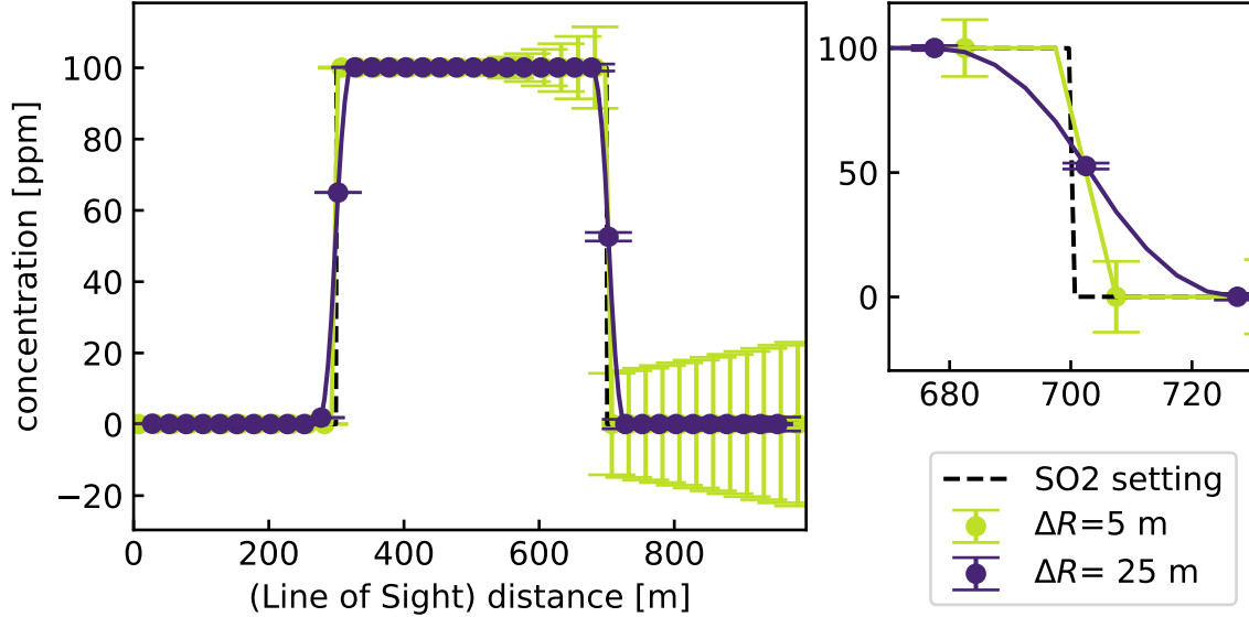
図 3.2: \Delta R = 5, 25\text{m} による \text{SO}_2 測定シミュレーション
