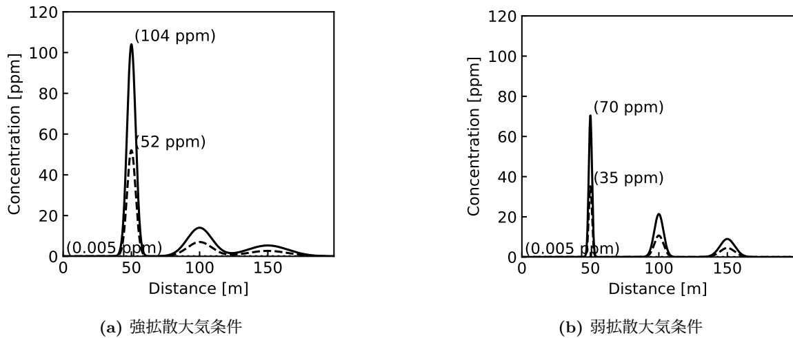
図 4.4: 大気拡散条件の違いによるライダー視線上の濃度分布設定
