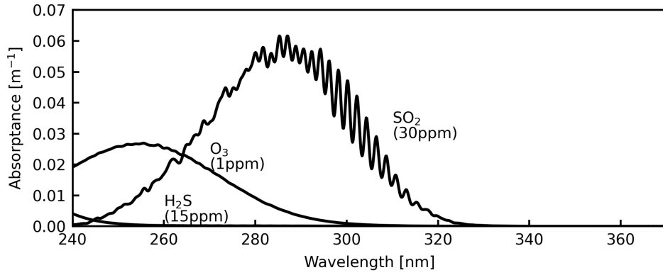
図 2.1: SO 2 , O 3 , H 2 S の吸収スペクトル
