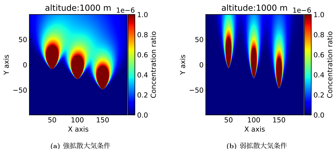
図 4.3: 大気拡散条件の違いによる地表面火山ガス分布
