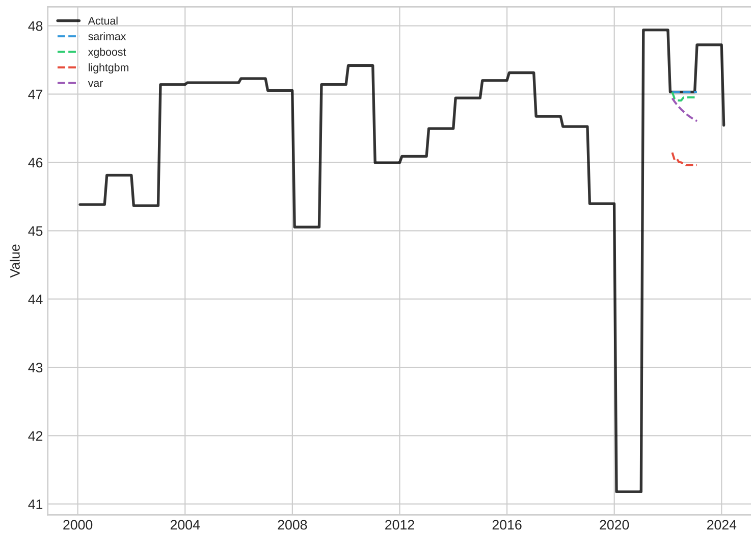
All Model Forecasts vs Actual
