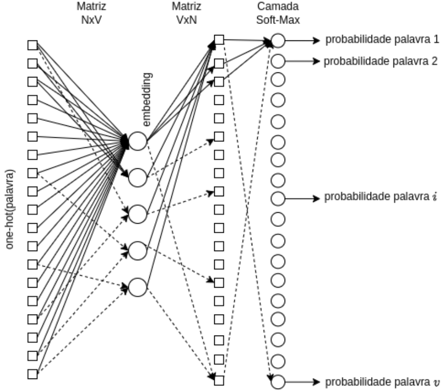
Figura 7: Processo de obtenção de embedding usando word2vec.
