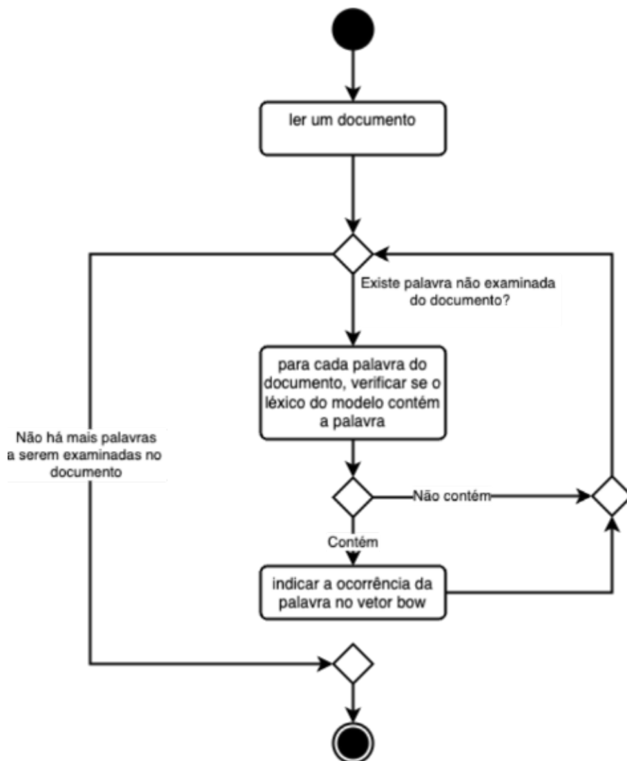
Figura 4: Algoritmo de extração de características para o BOW
