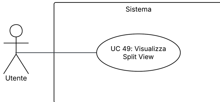
Figura 53: UC 49 – Visualizzazione Split View
