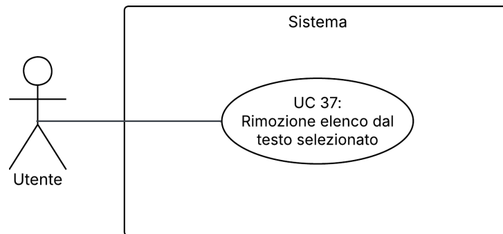
Figura 40: UC 37 – Rimozione formattazione elenco da testo selezionato
