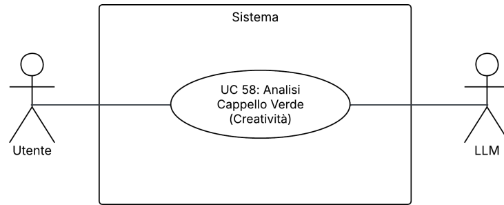
Figura 70: UC58 – Analisi Cappello Verde (Creatività)
