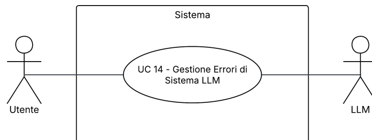
Figura 32: UC14 – Gestione errori di sistema LLM
