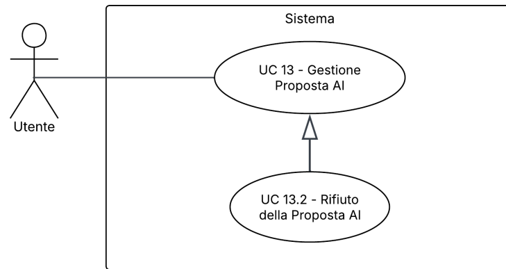
Figura 31: UC13.2 – Rifiuto della proposta AI
