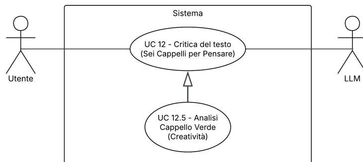
Figura 27: UC12.5 – Analisi Cappello Verde (Creatività)
