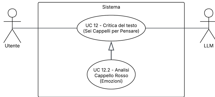
Figura 24: UC12.2 – Analisi Cappello Rosso (Emozioni)
