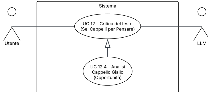
Figura 26: UC12.4 – Analisi Cappello Giallo (Opportunità)
