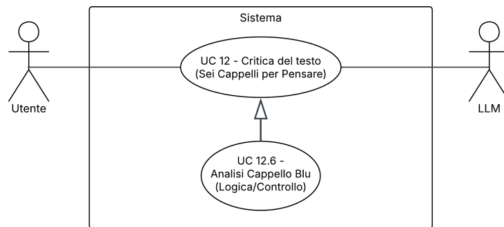
Figura 28: UC12.6 – Analisi Cappello Blu (Logica/Controllo)
