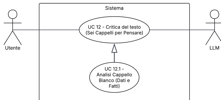
Figura 23: UC12.1 – Analisi Cappello Bianco (Dati e fatti)
