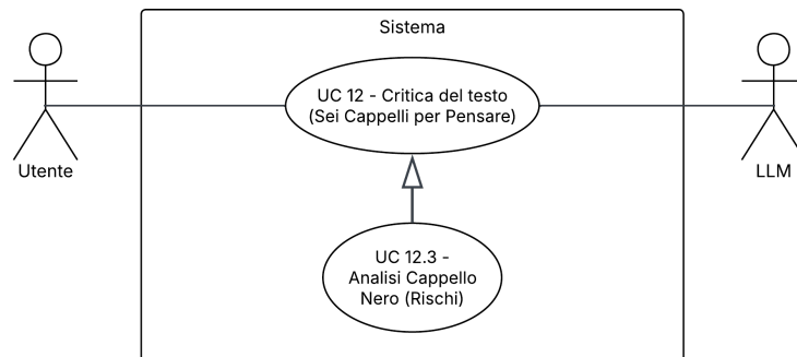
Figura 25: UC12.3 – Analisi Cappello Nero (Rischi)
