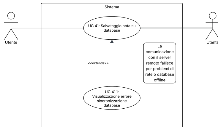
Figura 76: UC41.1 – Visualizzazione errore sincronizzazione Database
