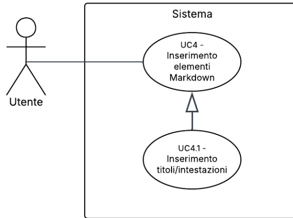
Figura 9: UC4 – Inserimento elementi Markdown
