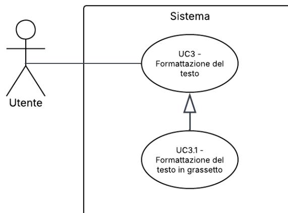
Figura 4: UC3.1 – Formattazione del testo in grassetto
