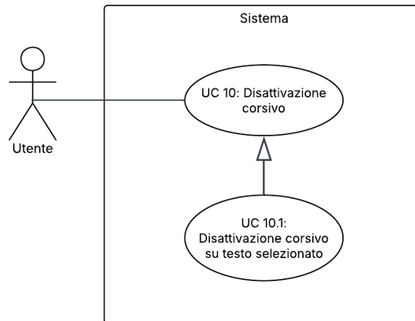
Figura 17: UC10.1 – Disattivazione corsivo su testo selezionato
