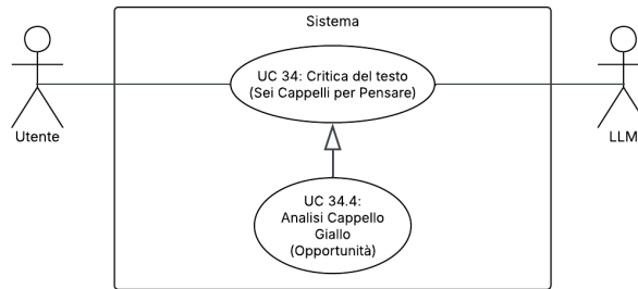
Figura 58: UC34.4 – Analisi Cappello Giallo (Opportunità)
