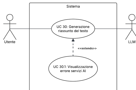
Figura 47: UC30.1 – Visualizzazione errore servizi AI
