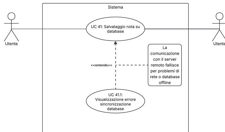
Figura 72: UC41.1 – Visualizzazione errore sincronizzazione Database
