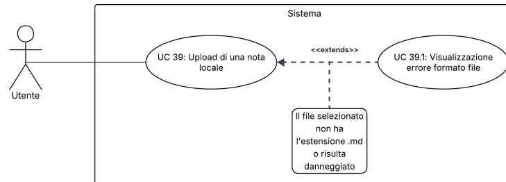
Figura 68: UC39.1 – Visualizzazione errore formato file
