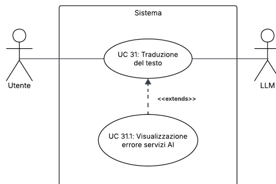
Figura 49: UC31.1 – Visualizzazione errore servizi AI
