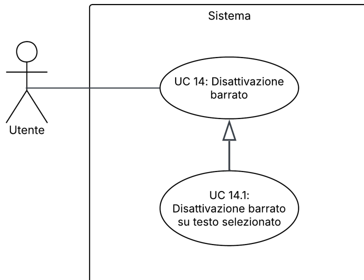
Figura 25: UC14.1 – Disattivazione barrato su testo selezionato
