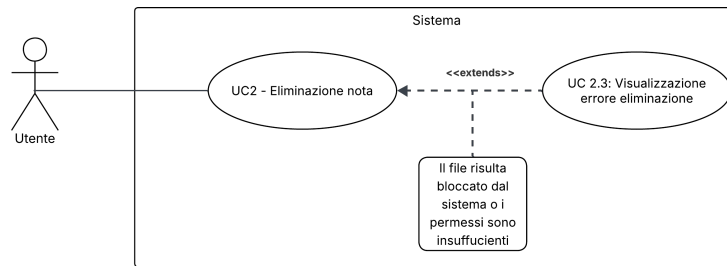
Figura 5: UC2.3 – Visualizzazione errore eliminazione
