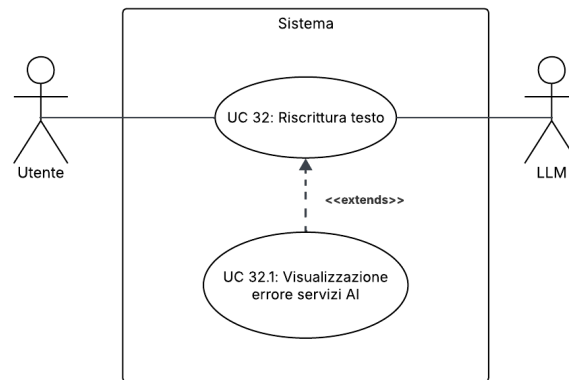
Figura 51: UC32.1 – Visualizzazione errore servizi AI
