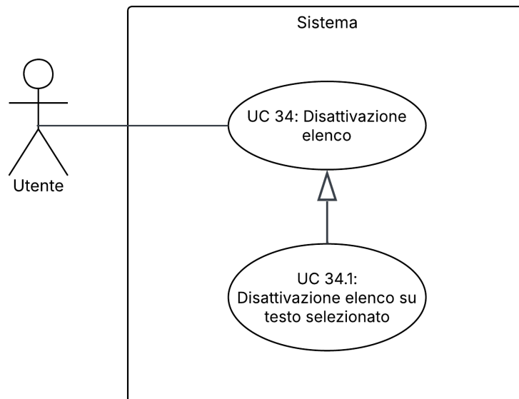
Figura 40: UC 34.1 – Disattivazione elenco su testo selezionato
