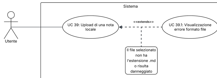
Figura 68: UC39.1 – Visualizzazione errore formato file
