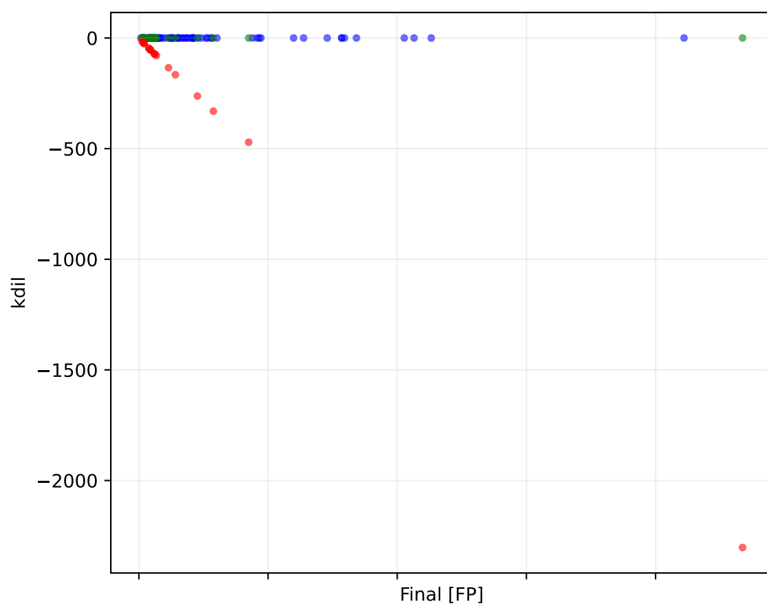
PIAE Epoch 0 lambda physics 0.0000
