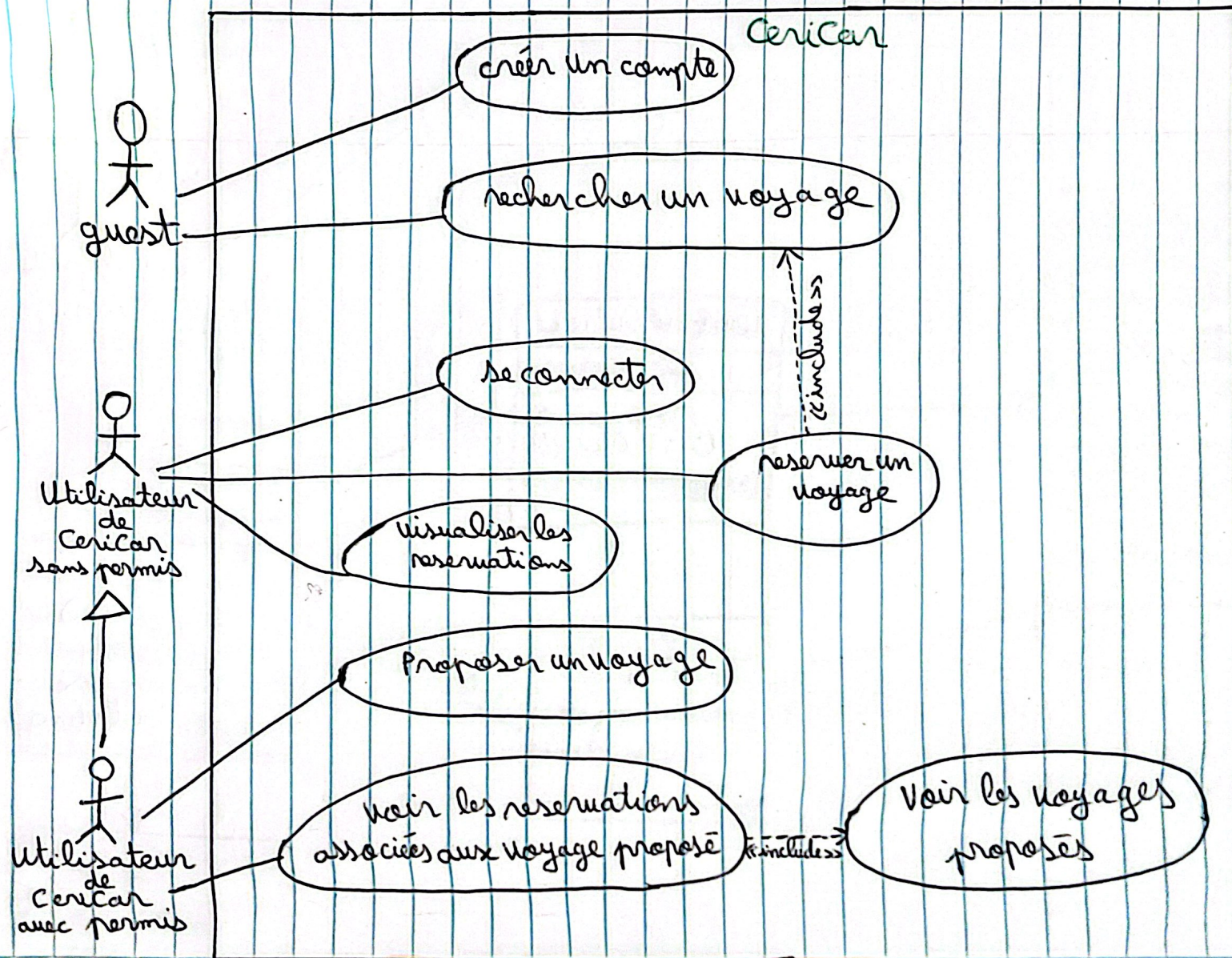
Diagramme de cas d'utilisation de CeriCar
