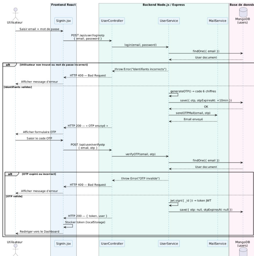
Figure III.3 : Diagramme de séquence objet du cas d'utilisation « Se connecter avec OTP »
