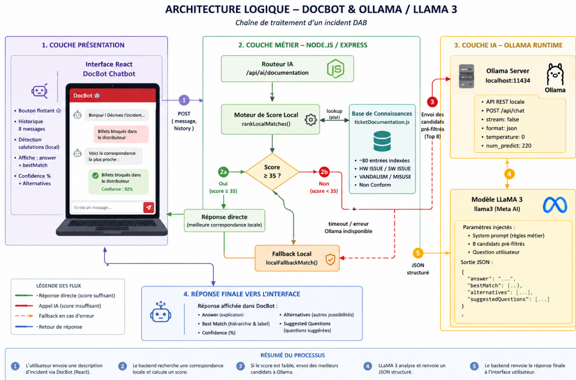
Figure IV.5 : Architecture logique du module DocBot basé sur Ollama
