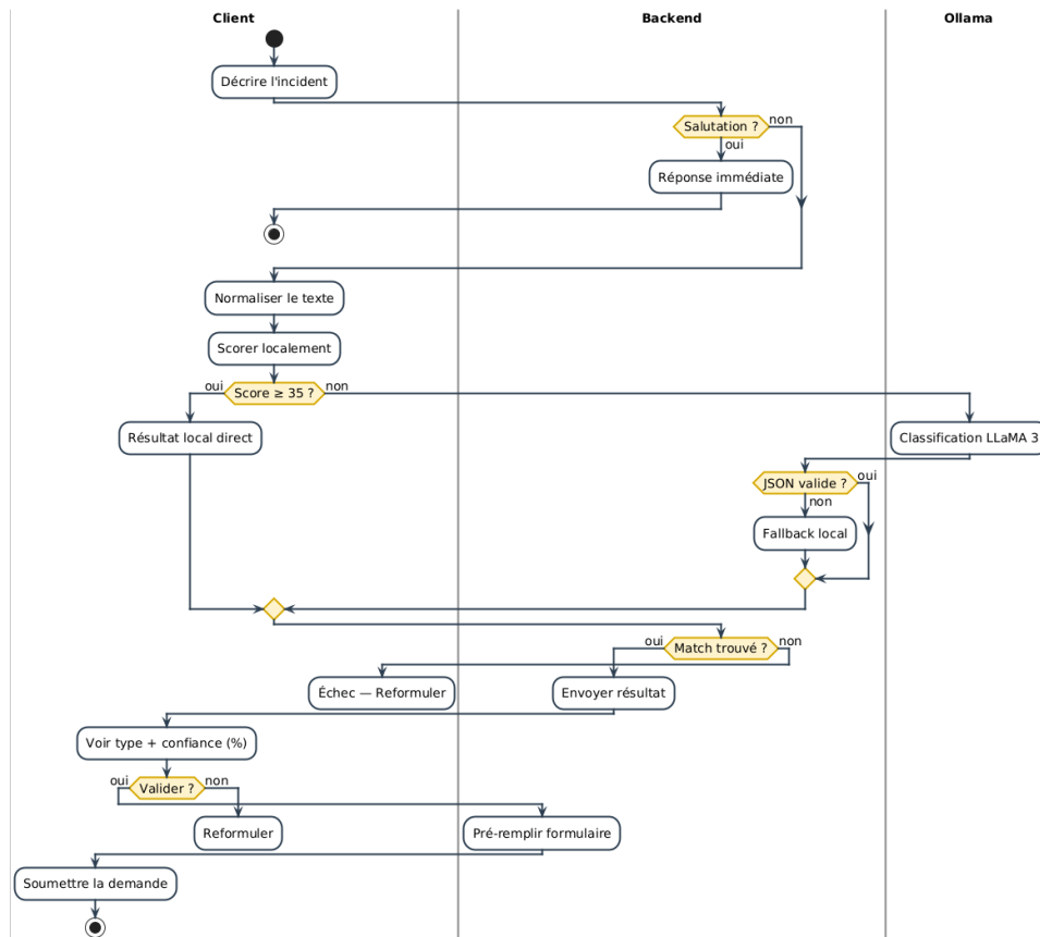
Figure IV.8 : Diagramme d'activités - Identification d'un incident via DocBot
