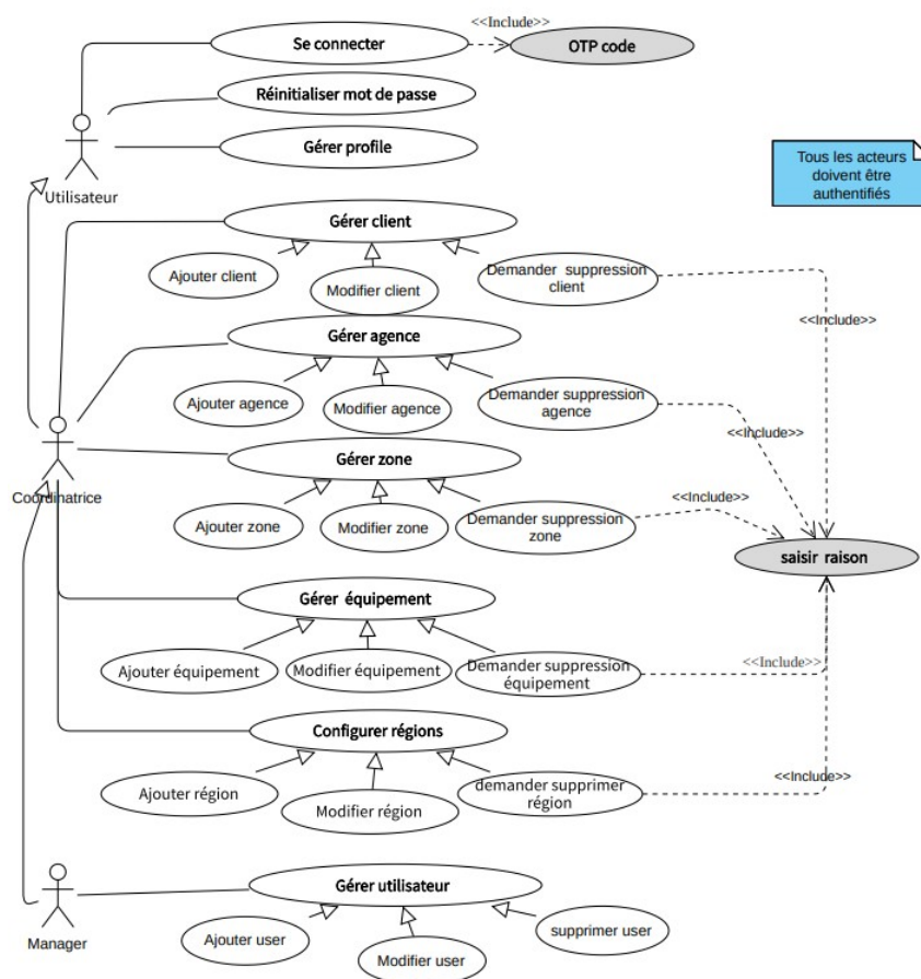
Figure III.1 : Diagramme de cas d'utilisation du Sprint 1
