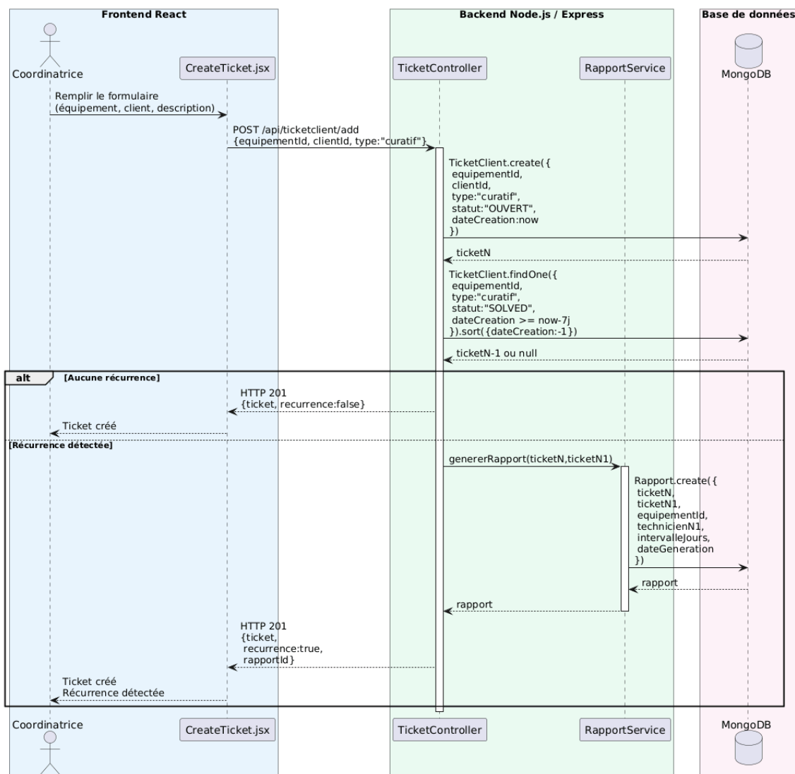
Figure V.3 : Diagramme de séquence objet — Détecter une récurrence et générer un rapport
