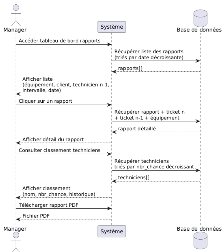
Figure V.4 : Diagramme de séquence système — Consulter le tableau de bord des rapports
