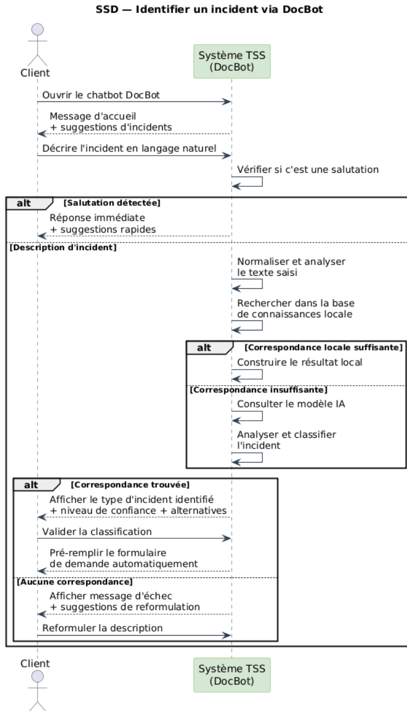
Figure IV.6 : Diagramme de séquence système - DocBot
