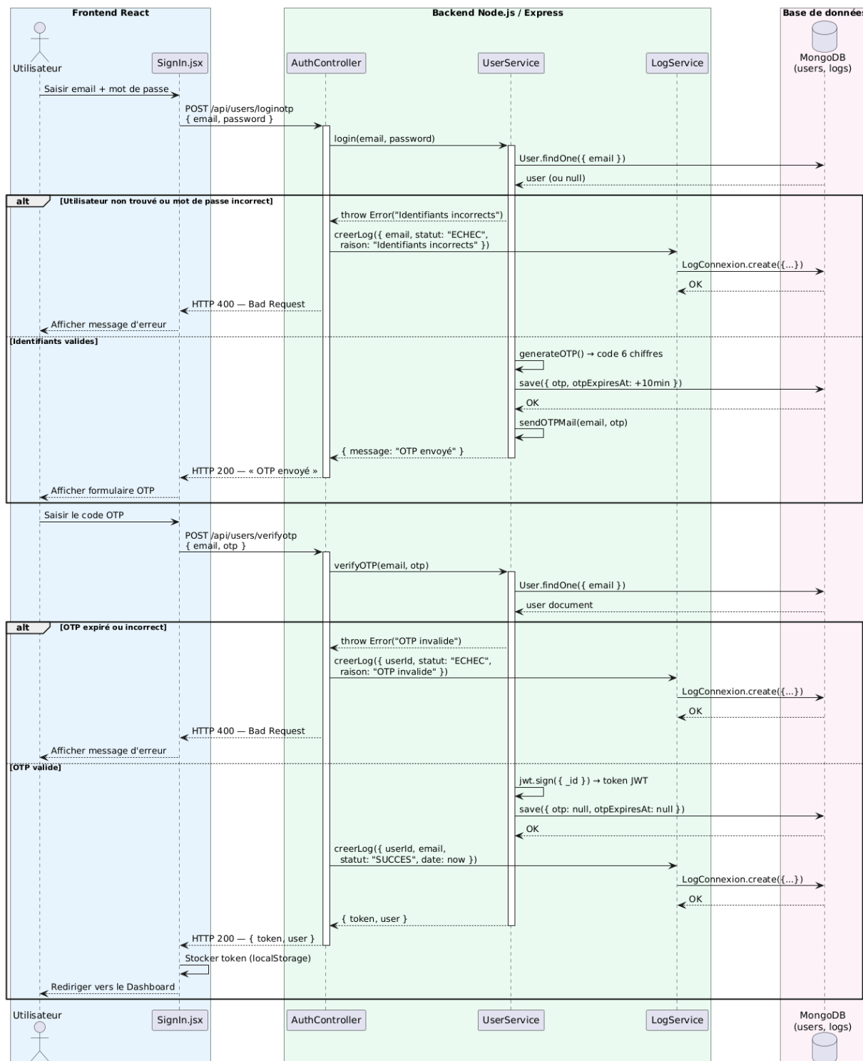
Figure VI.3 : Diagramme de séquence objet — Enregistrer un log de connexion
