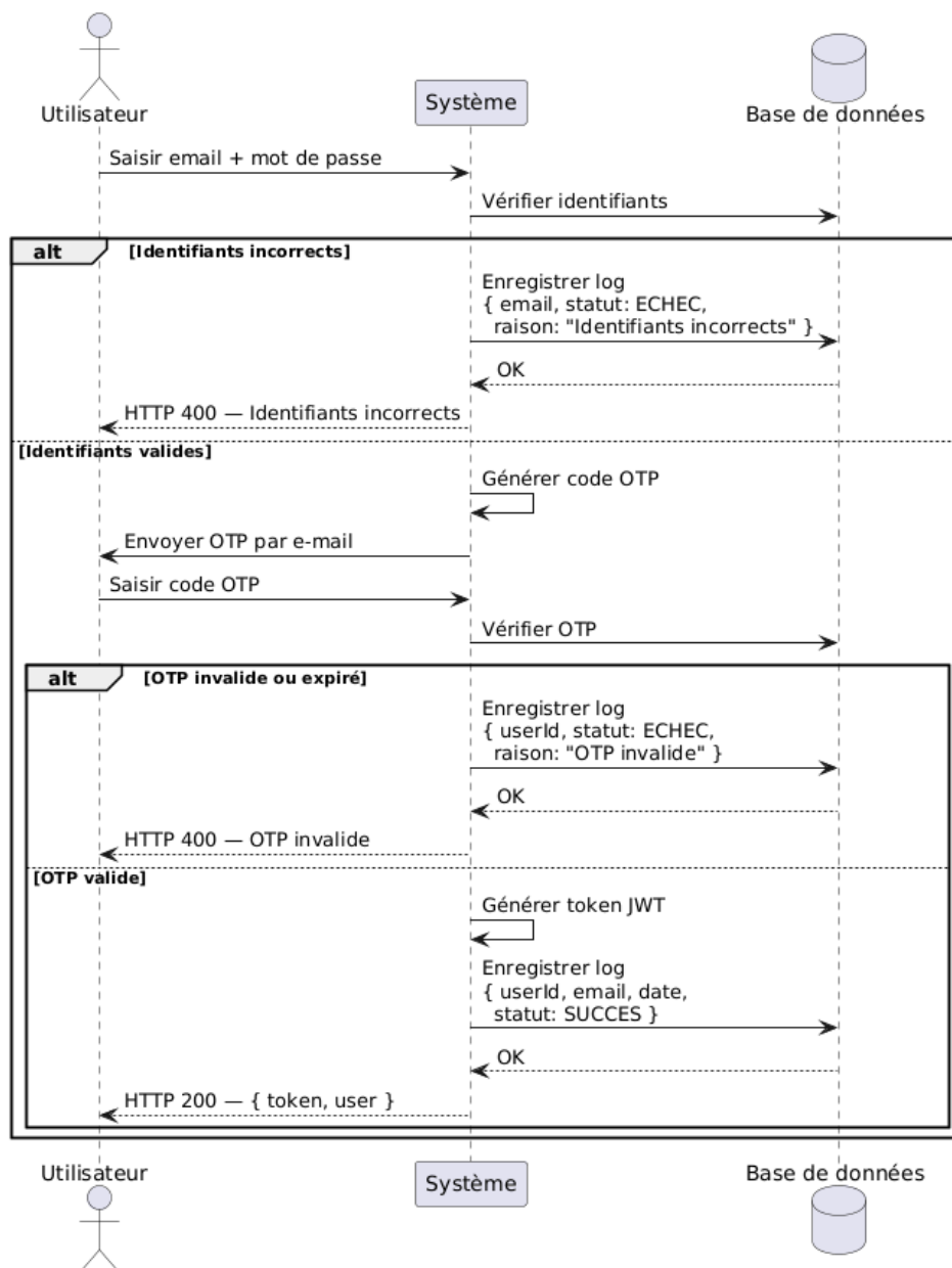
Figure VI.2 : Diagramme de séquence système — Enregistrer un log de connexion
