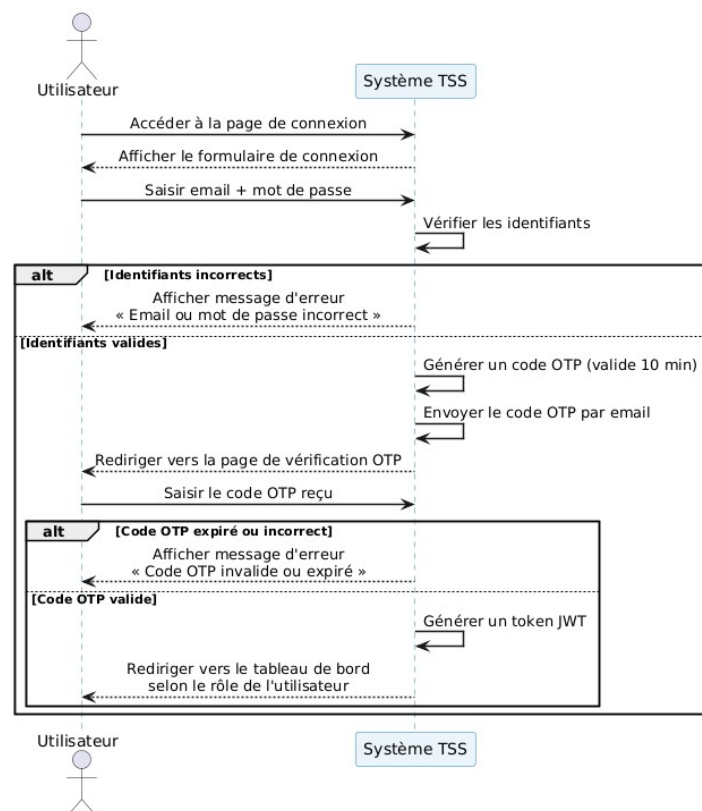
Figure III.2 : Diagramme de séquence système du cas d'utilisation « Se connecter avec OTP »
