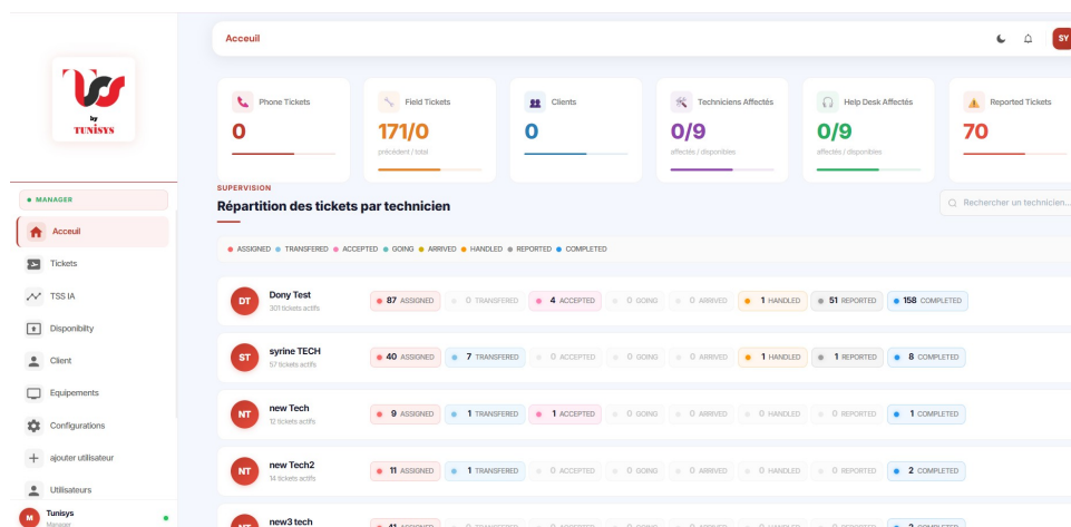
Figure III.16 : Tableau de bord
