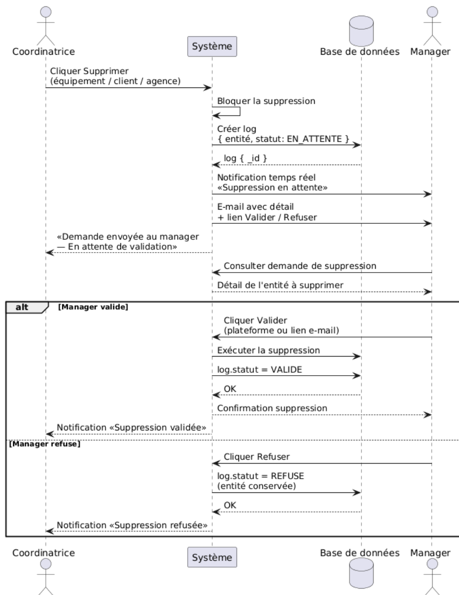
Figure VI.6 : Diagramme de séquence système — Valider une suppression
