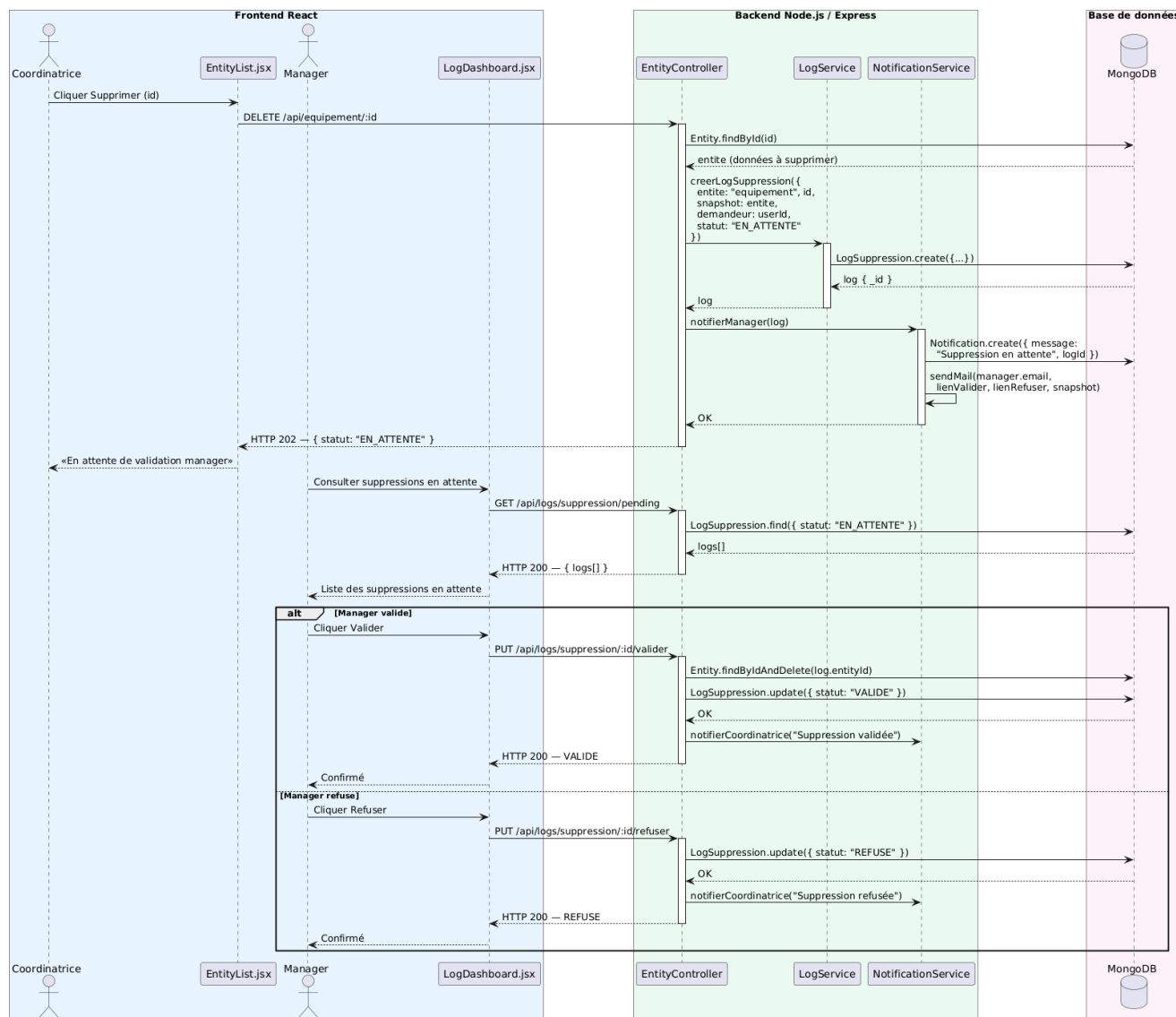
Figure VI.7 : Diagramme de séquence objet — Valider une suppression
