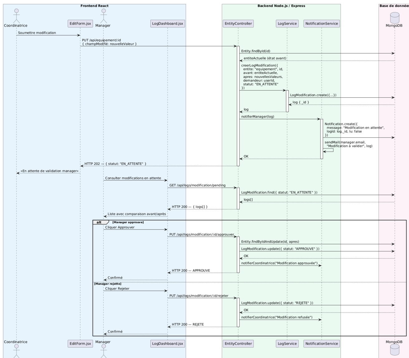
Figure VI.5 : Diagramme de séquence objet — Valider une modification
