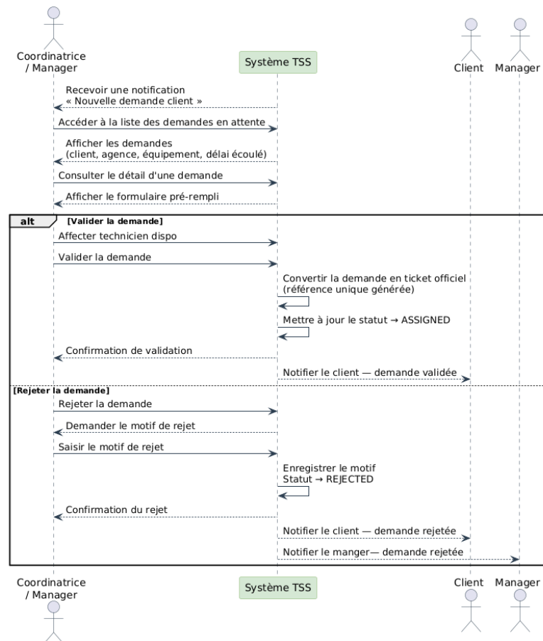
Figure IV.2 : Diagramme de séquence système du « Traitement d'une demande par la Coordinatrice »
