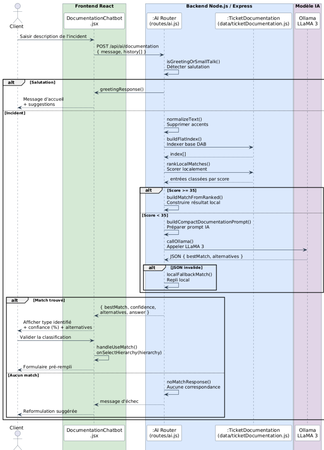
Figure IV.7 : Diagramme de séquence objet - DocBot
