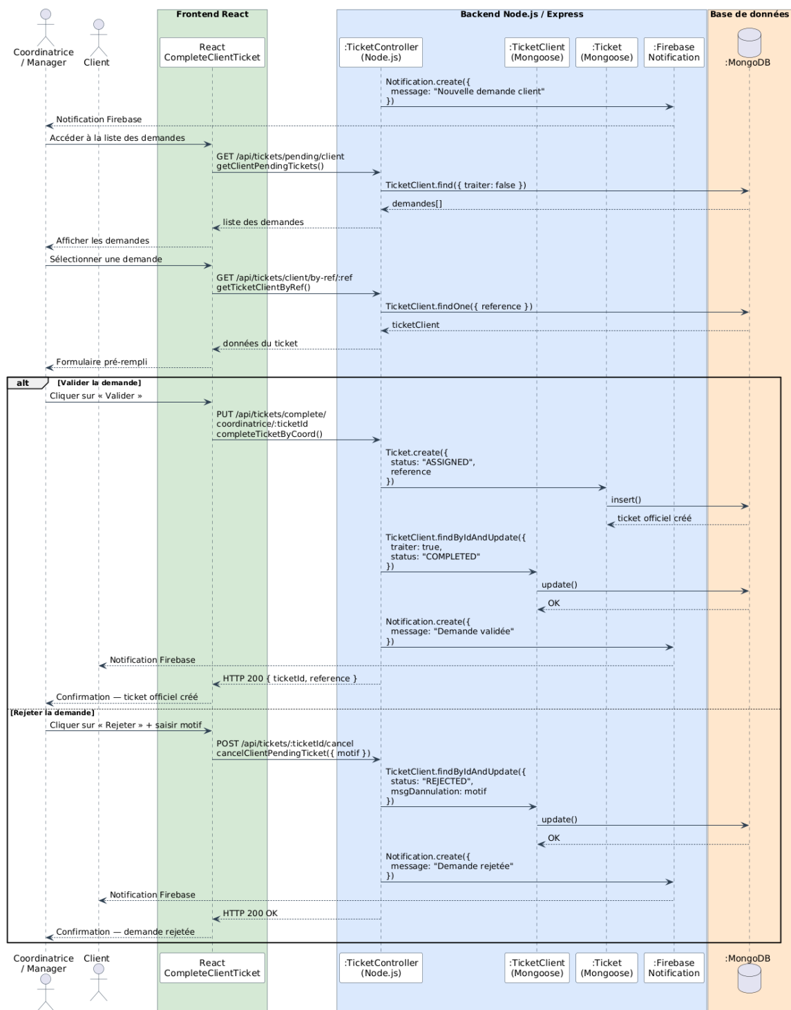
Figure IV.3 : Diagramme de séquence objet « Traitement d'une demande par la Coordinatrice »
