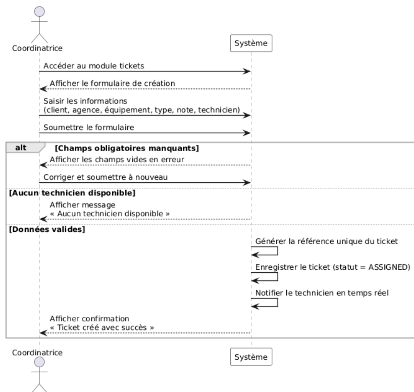
Figure III.11 : Diagramme de séquence système « Ajouter un ticket »
