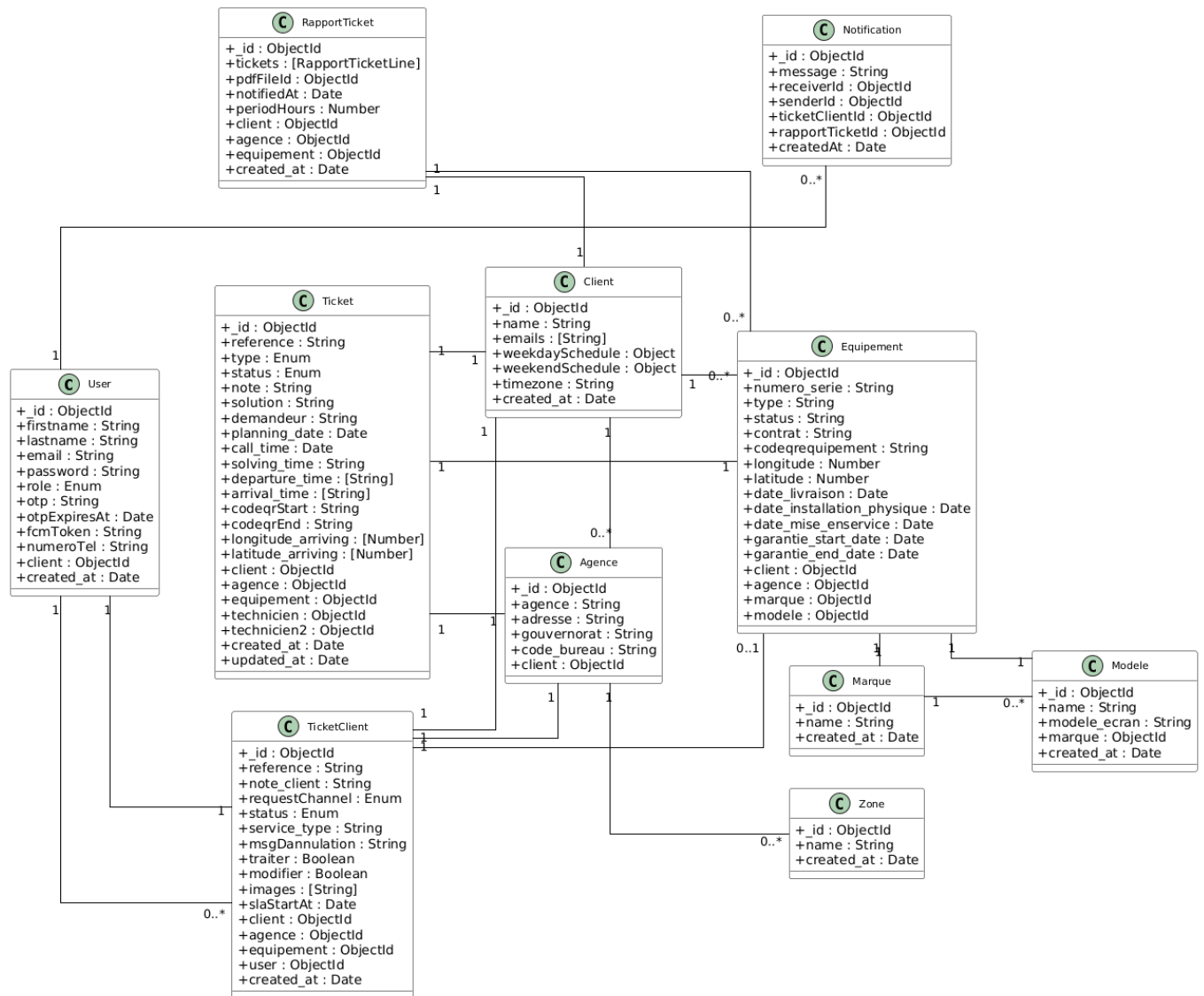
FIGURE II.2 : Diagramme de classe d'analyse Global.
