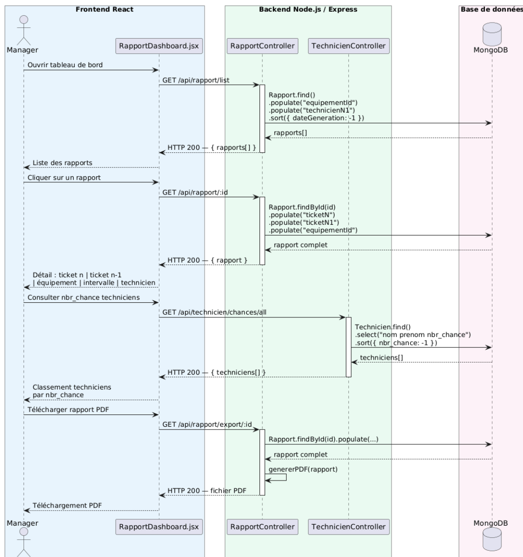
Figure V.5 : Diagramme de séquence objet — Consulter le tableau de bord des rapports
