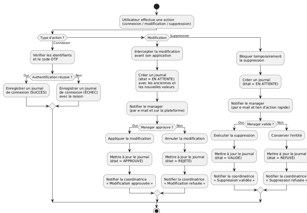
Figure VI.8 : Diagramme d'activité — Sprint 5 : Logs et validation manager
