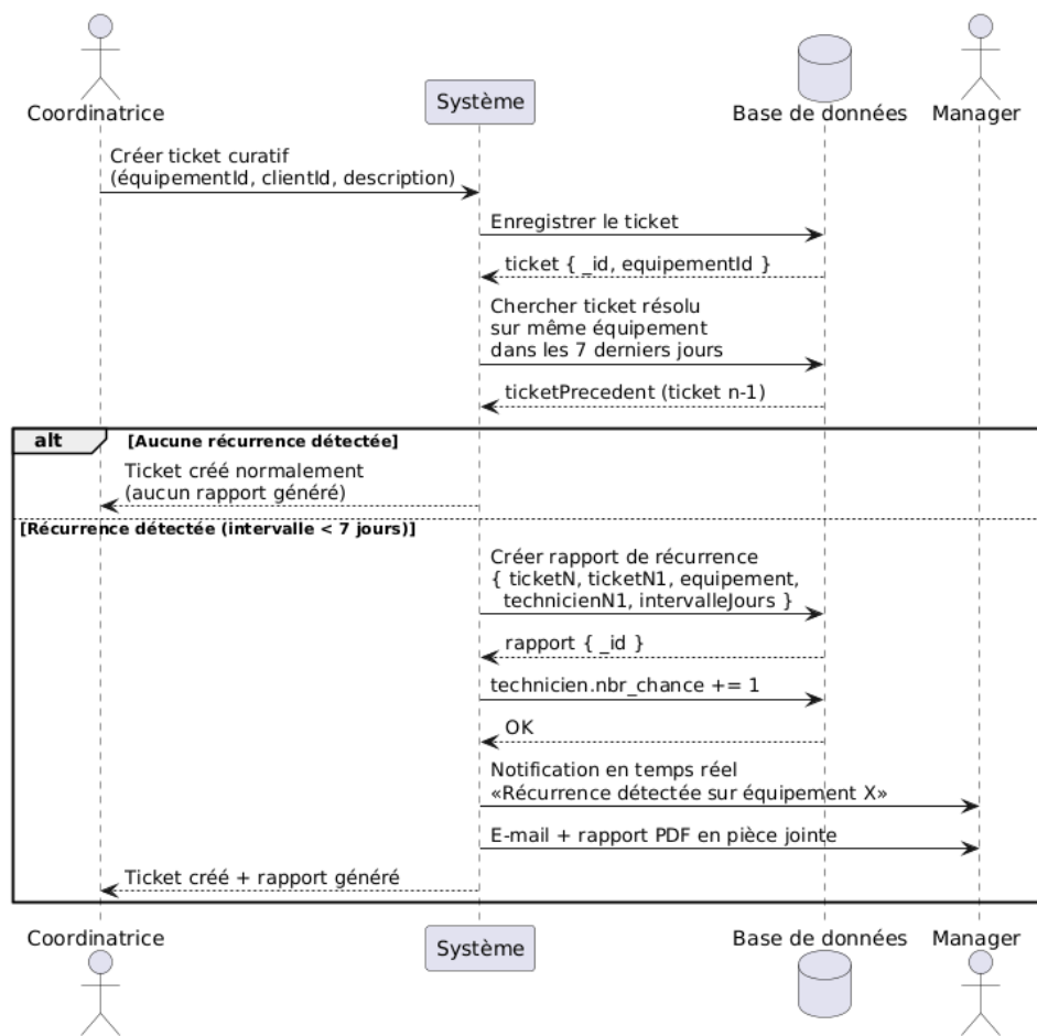
Figure V.2 : Diagramme de séquence système — Détecter une récurrence et générer un rapport
