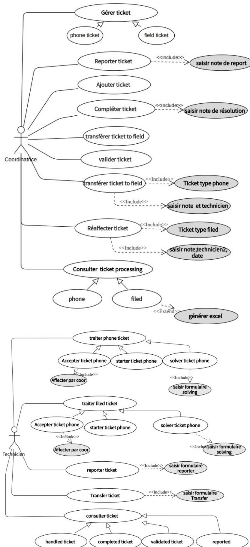
Figure III.10 : Diagramme de cas d'utilisation du Sprint 2
