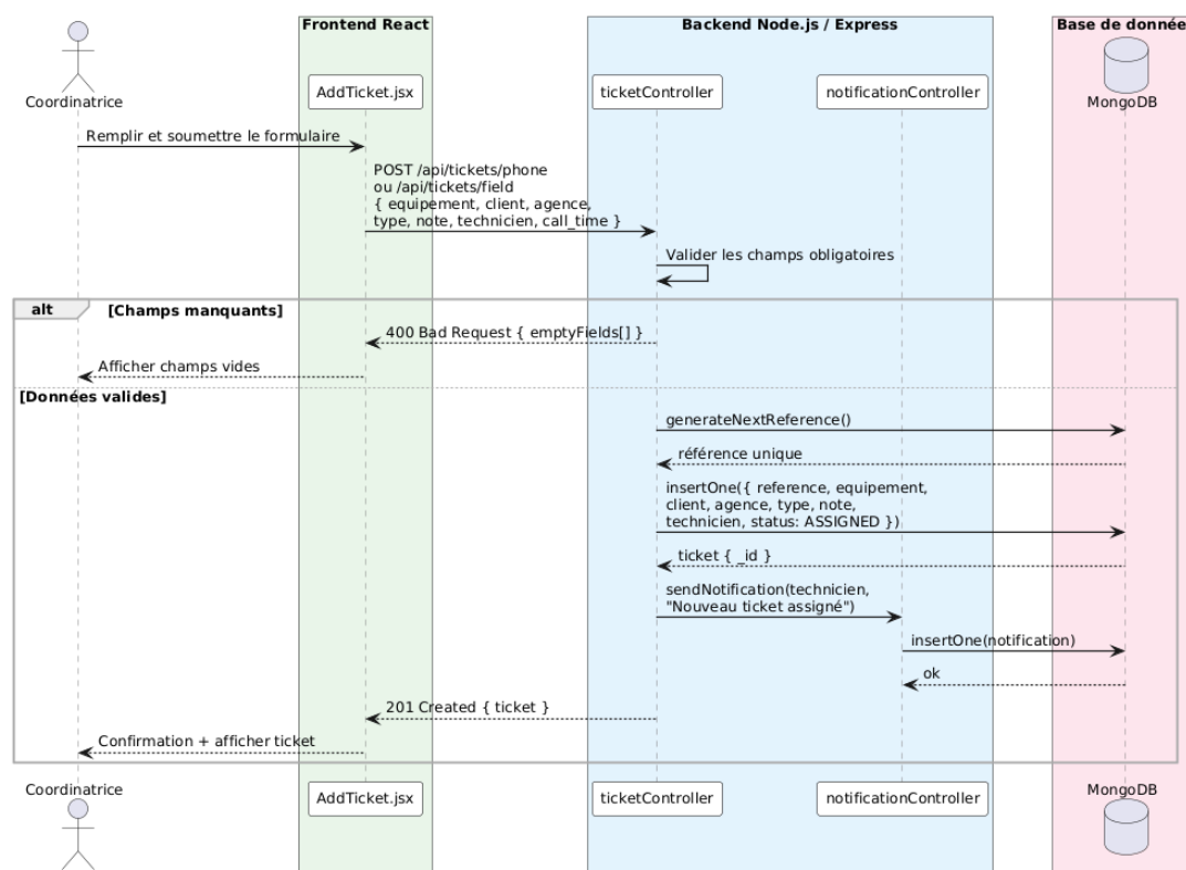
Figure III.12 : Diagramme de séquence objet « Ajouter un ticket »
