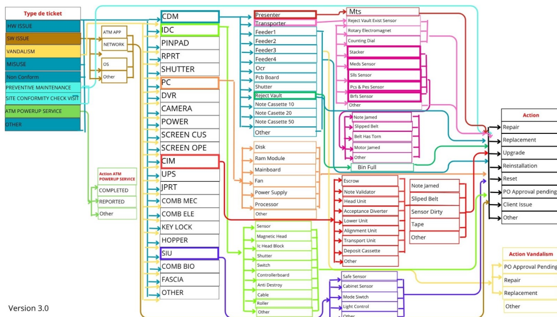
Figure IV.4 : Classification des incidents des DAB selon la documentation TUNISYS
