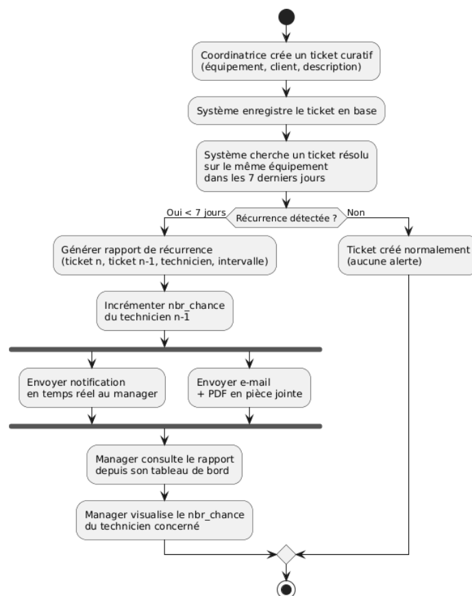
Figure V.6 : Diagramme d'activité — Sprint 4 : Détection de récurrence et alertes
