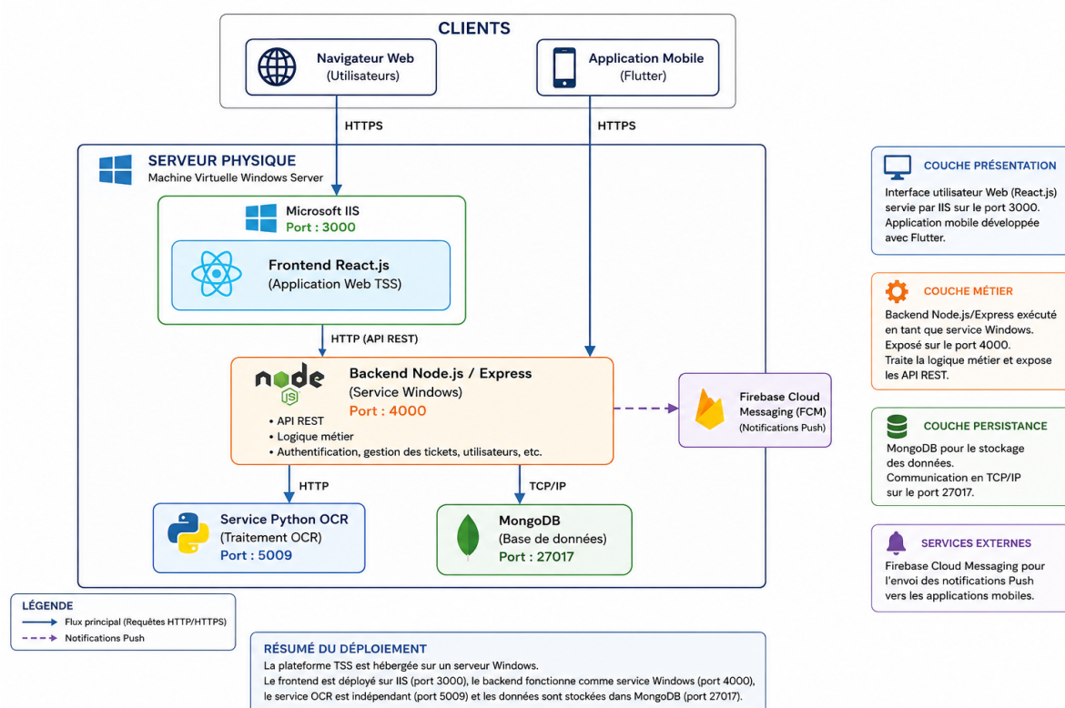
Figure II.4 : Architecture physique de la plateforme TSS.
