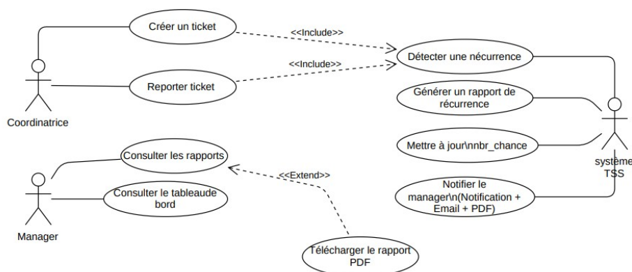
Figure V.1 : Diagramme de cas d'utilisation du Sprint 4
