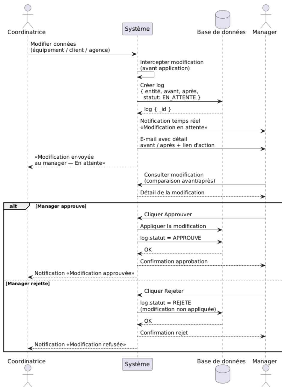
Figure VI.4 : Diagramme de séquence système — Valider une modification
