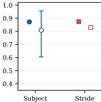
HD→PD / QDA
