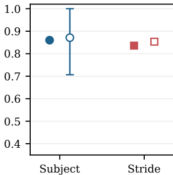
PD→HD / QDA
