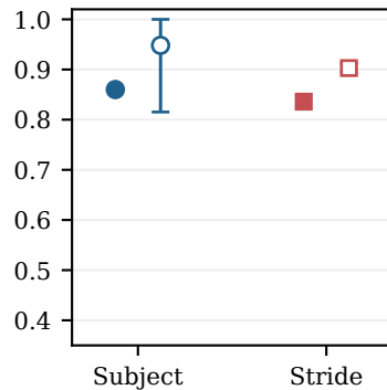
PD→ALS / QDA
