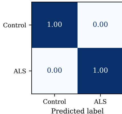
ALS / QDA
