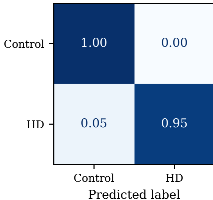
HD / XGBoost
