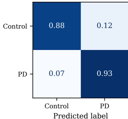
PD / DT
