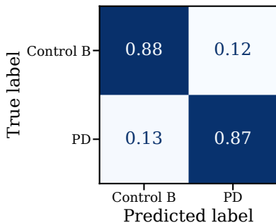
ALS→PD / DT
