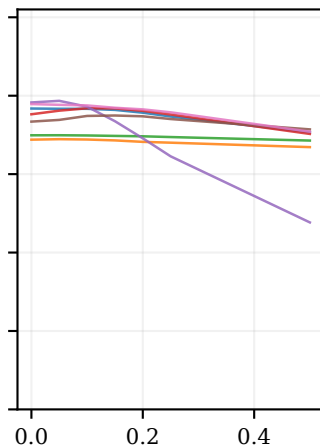
ALS→HD
