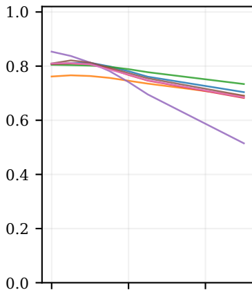
ALS→PD
