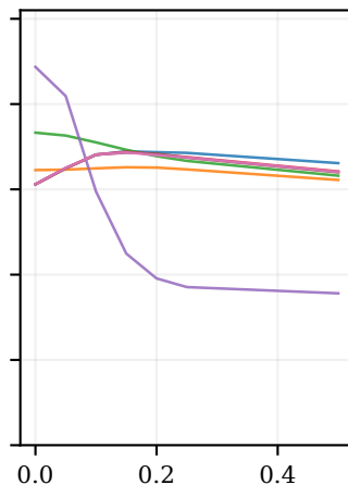
HD→ALS
