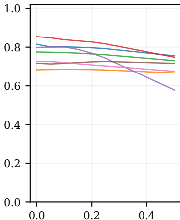
ALS→PD
