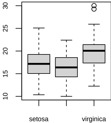
Sepal.Area
