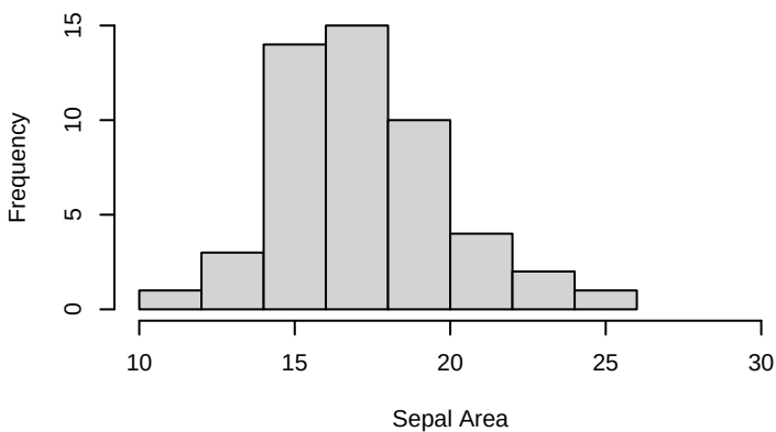
Iris setosa
