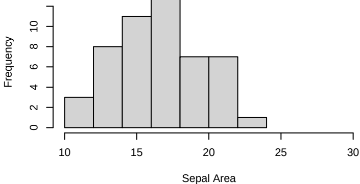
Iris virginica
