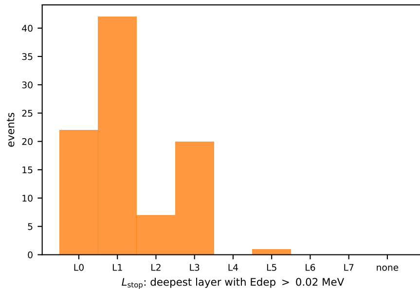
deuteron truth
