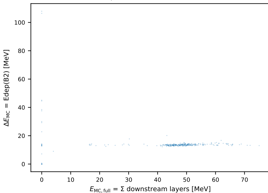
proton truth (n=313)
