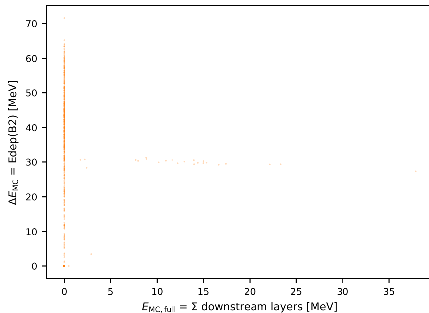
deuteron truth (n=790)
