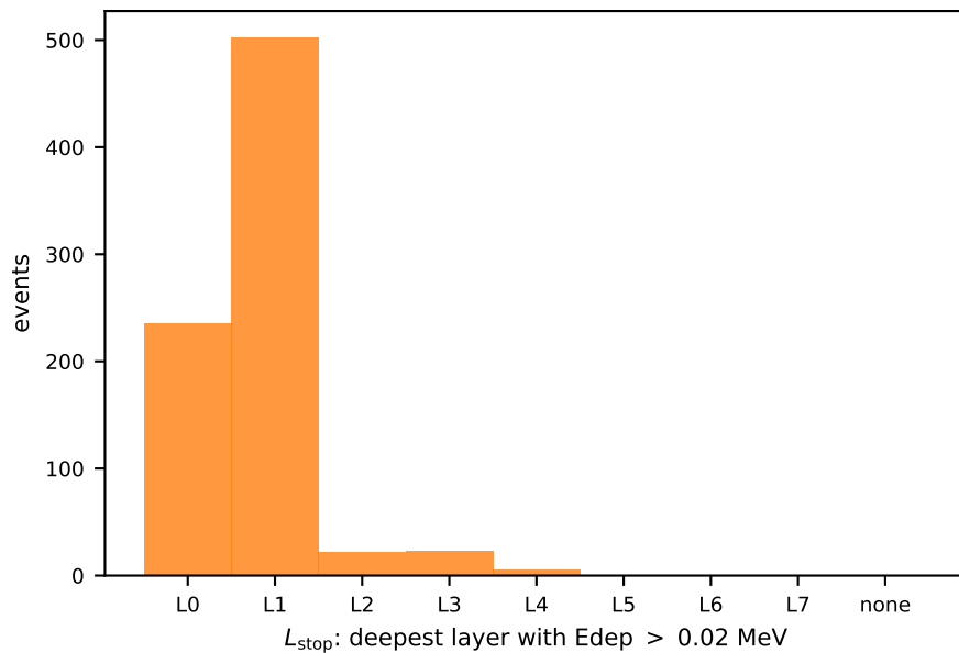
deuteron truth
