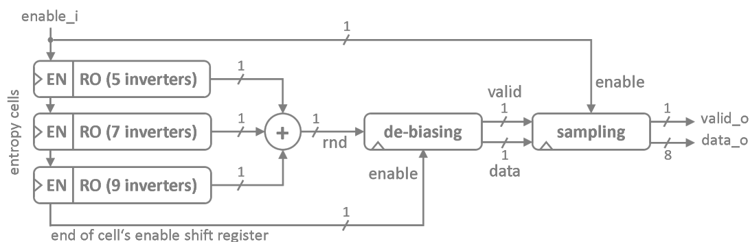
RYSUNEK 3.1: Model źródła entropii. [4]
