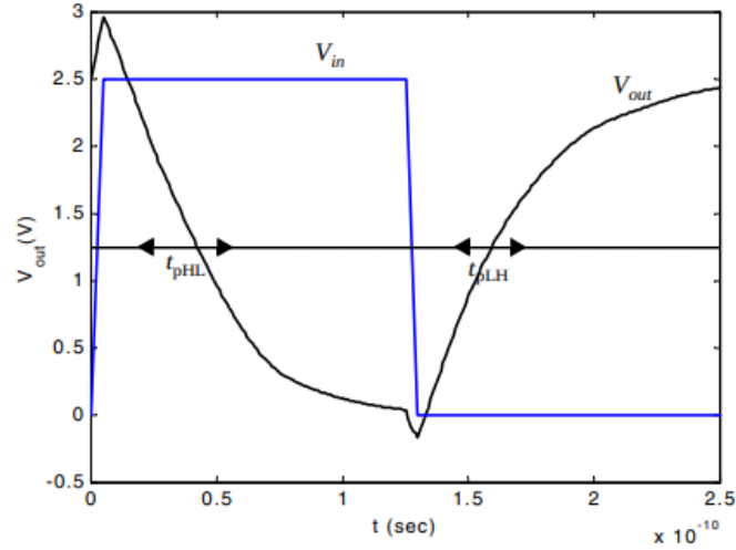
RYSUNEK 2.5: Propagacja sygnału wewnątrz inwertera CMOS - symulacja. [4]
