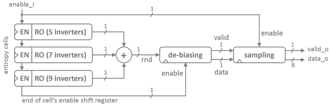
RYSUNEK 3.1: Architektura neoTRNG [5].
