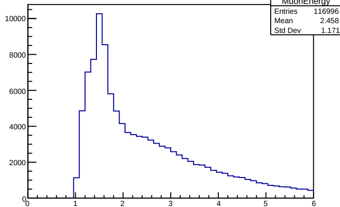
MuonEnergy
