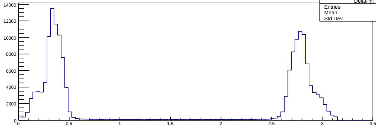
DeltaPhi
