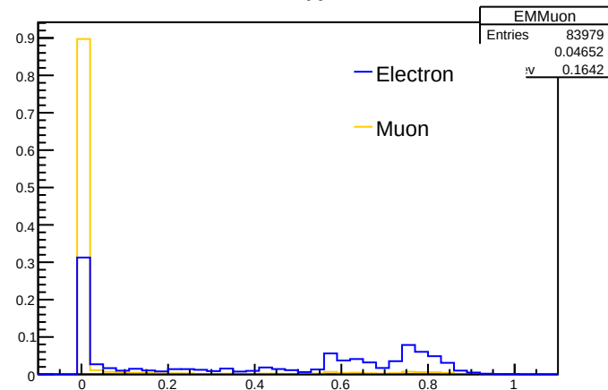
EMMuon
