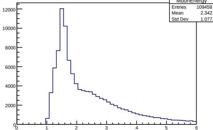
MuonEnergy
