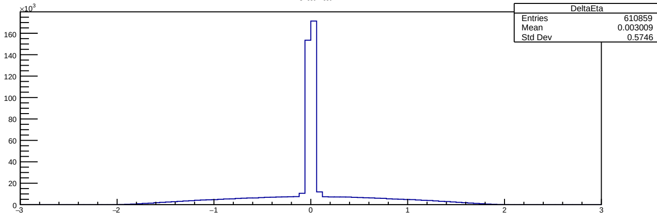
DeltaEta
