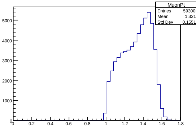
MuonPt
