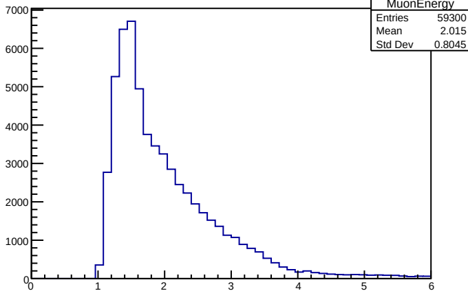
MuonEnergy
