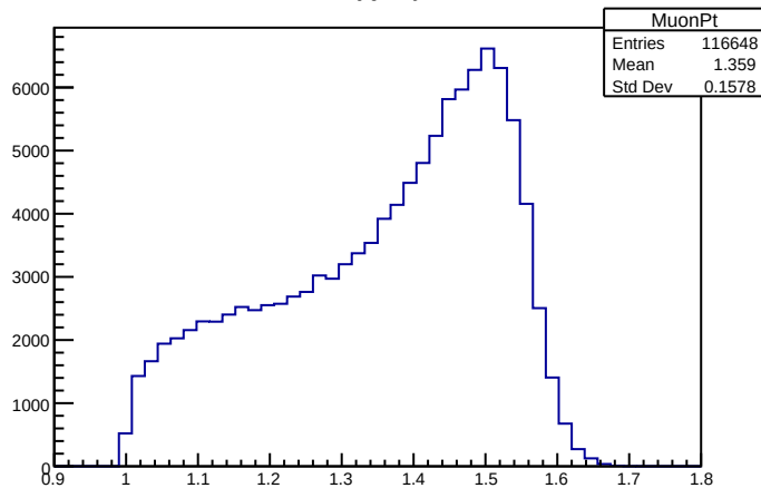
MuonPt
