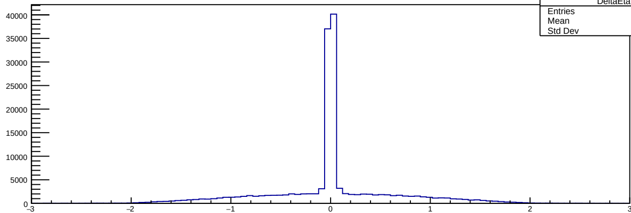
DeltaEta
