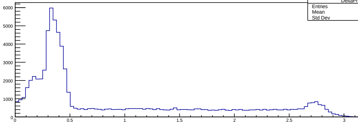
DeltaPhi
