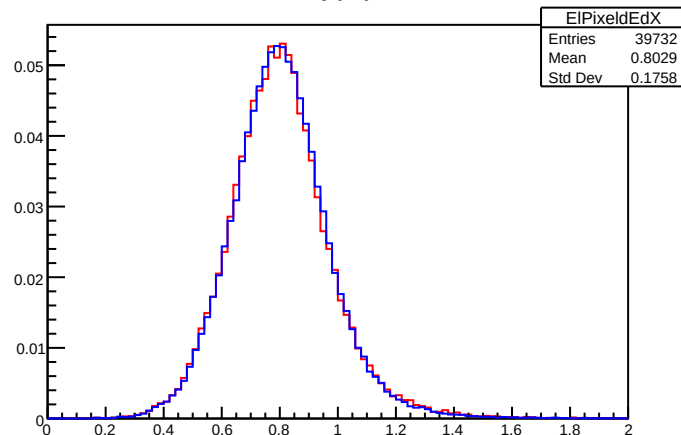
PixelEdX
