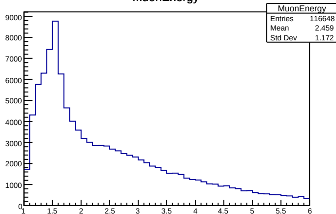
MuonEnergy
