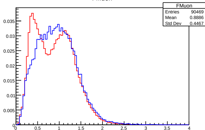
FMuon
