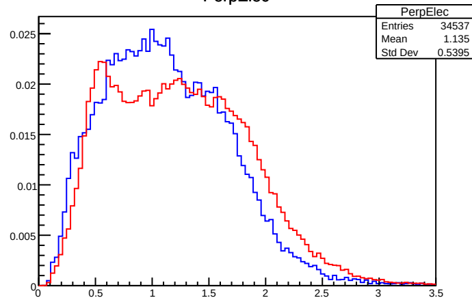
PerpElec
