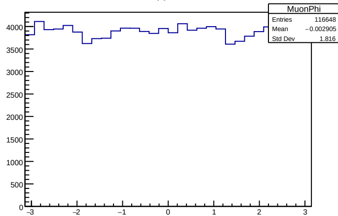
MuonPhi
