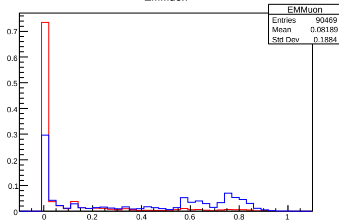
EMMuon
