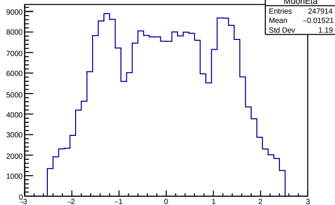
MuonEta
