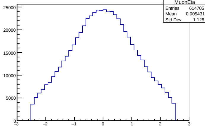
MuonEta
