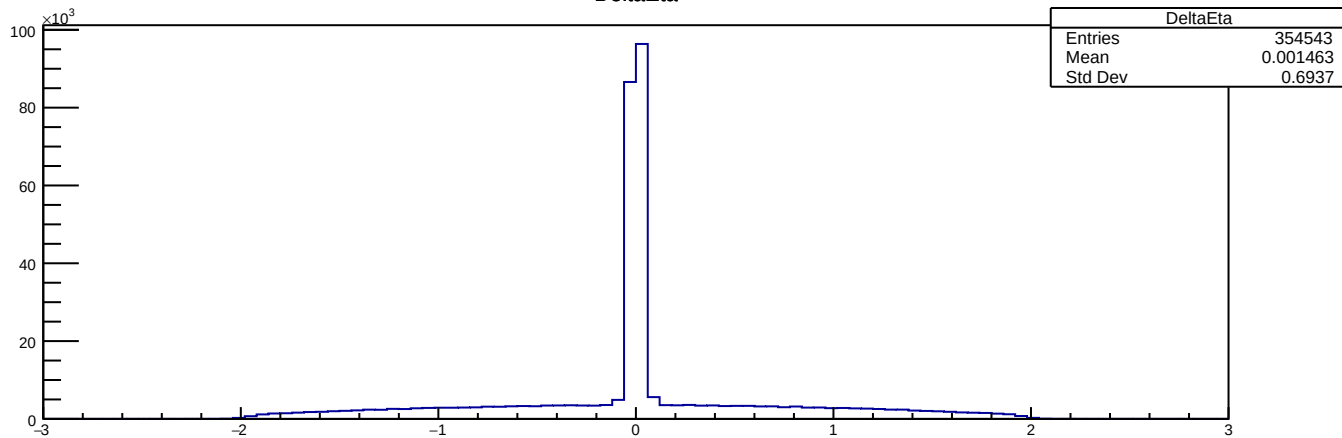
DeltaEta
