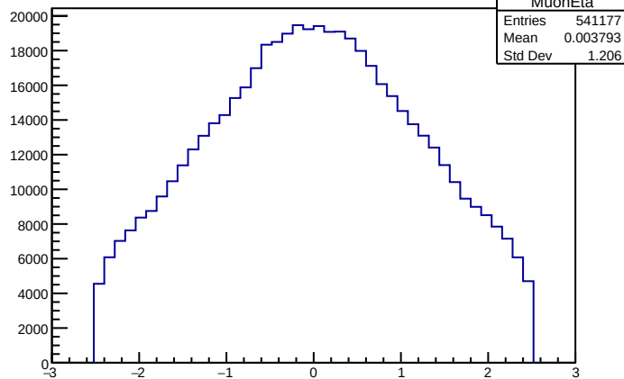
MuonEta
