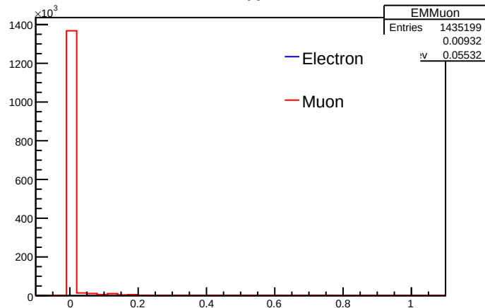
EMMuon
