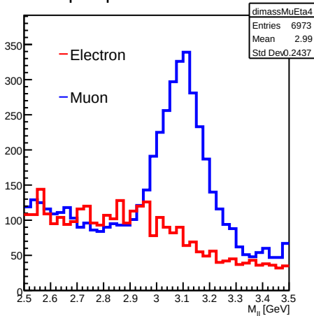
Lepton pair mass: Eta: 2 - 2.5
