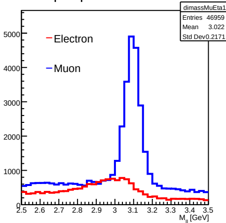
Lepton pair mass: Eta: 0.5 - 1
