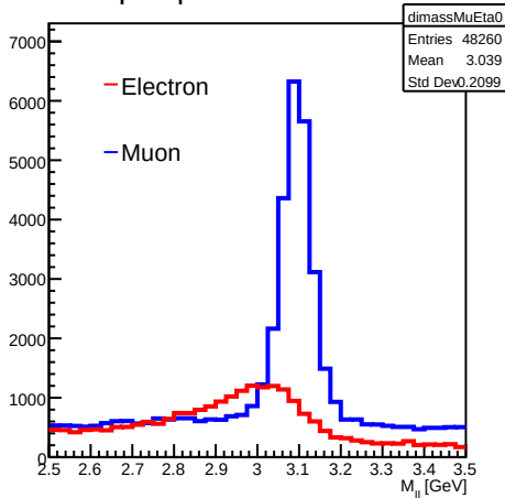
Lepton pair mass: Eta: 0 - 0.5
