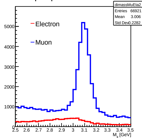
Lepton pair mass: Eta: 1 - 1.5
