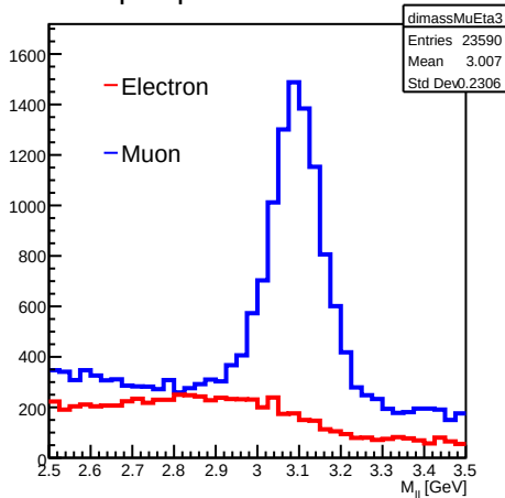
Lepton pair mass: Eta: 1.5 - 2
