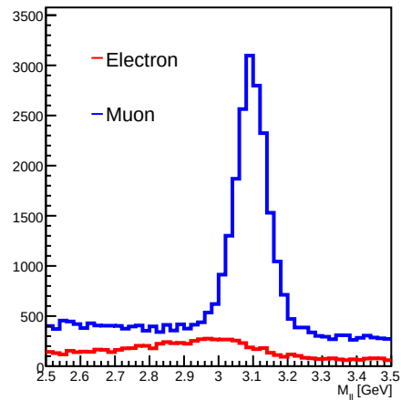
Lepton pair mass: Eta: 1 - 1.5
