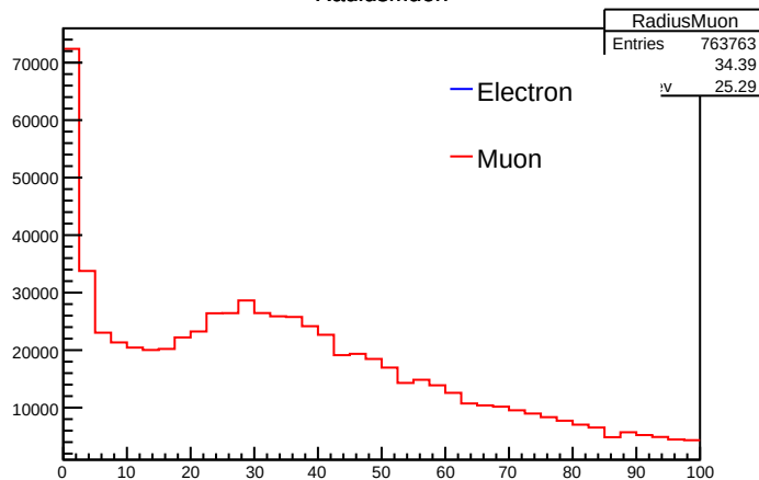
RadiusMuon
