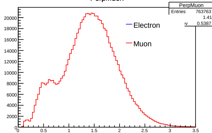
PerpMuon
