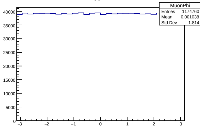
MuonPhi
