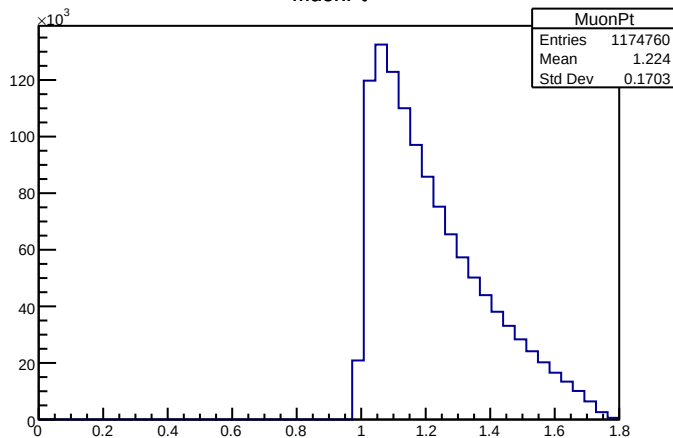
MuonPt
