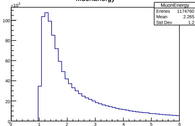
MuonEnergy
