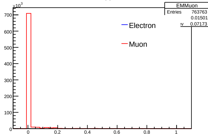
EMMuon
