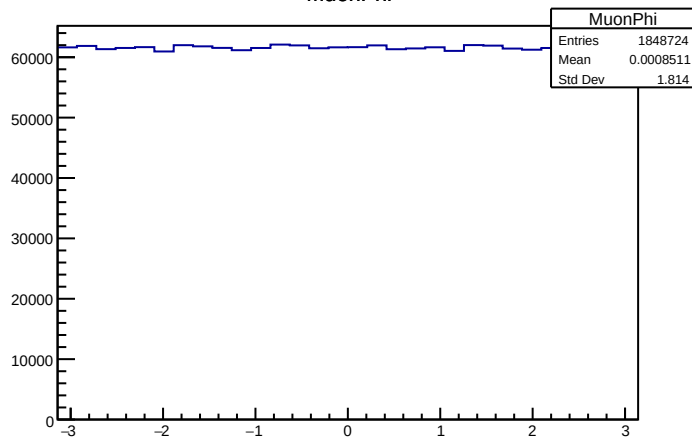
MuonsPhi
