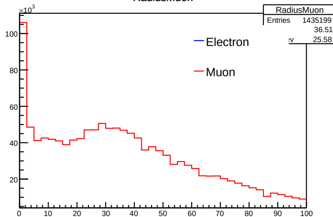
RadiusMuon
