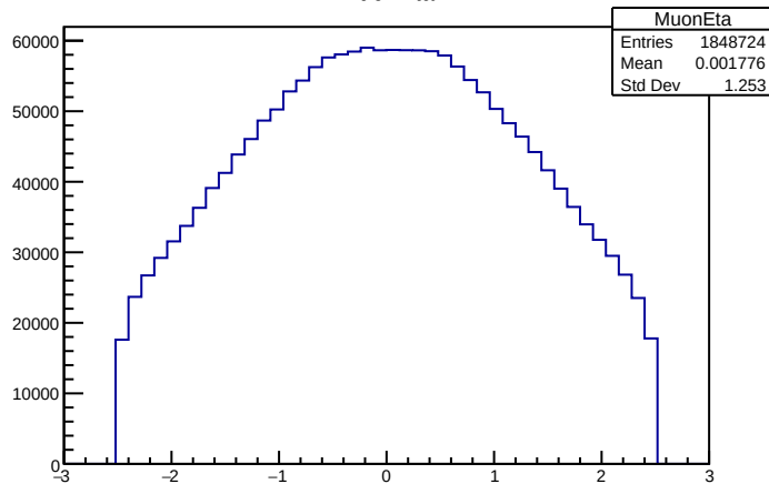
MuonsEta
