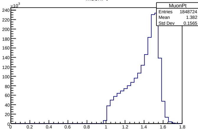
MuonsPt
