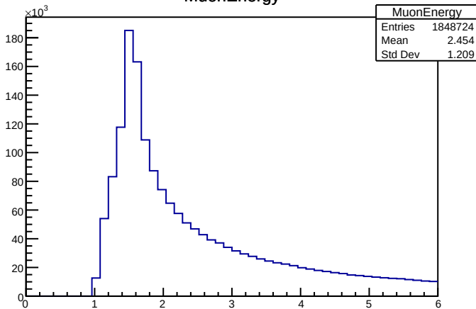
MuonsEnergy
