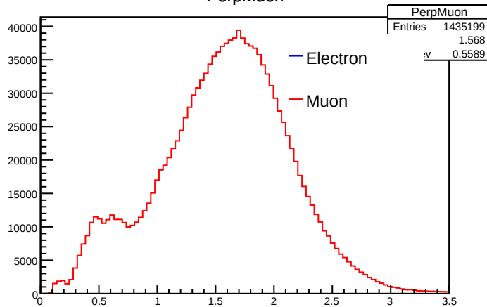
PerpMuon
