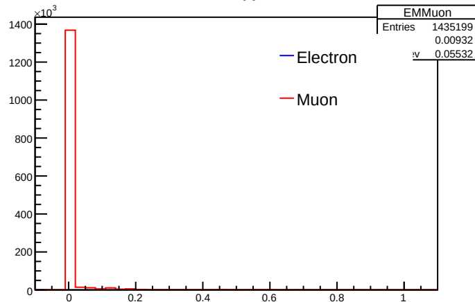
EMMuon
