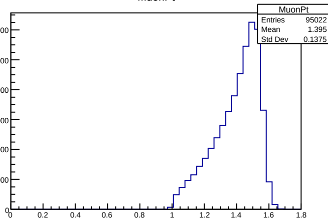
MuonPt
