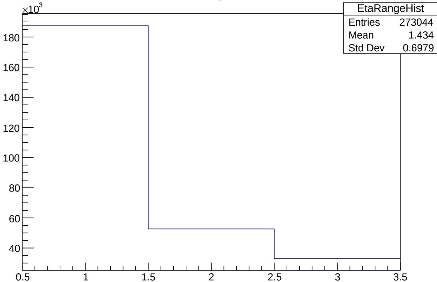
EtaRangeHist
