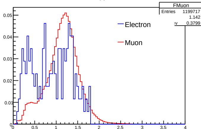
FMuon
