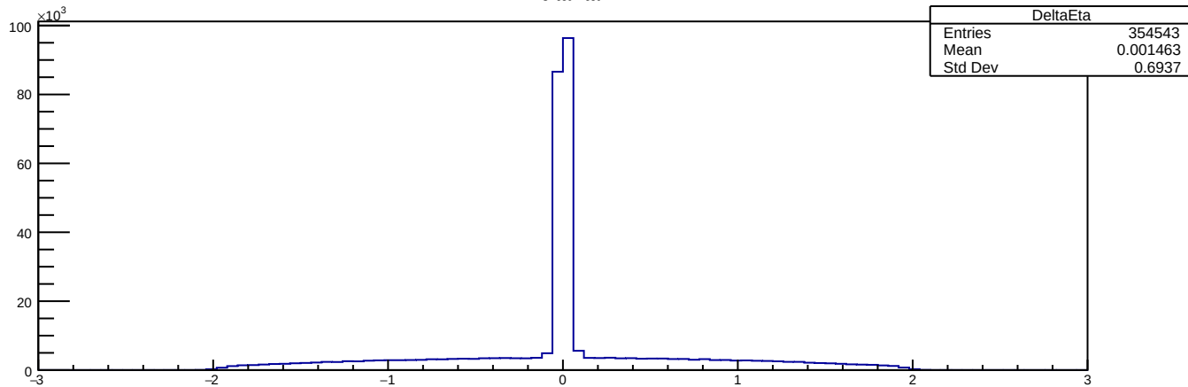
DeltaEta
