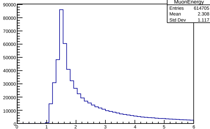
MuonEnergy
