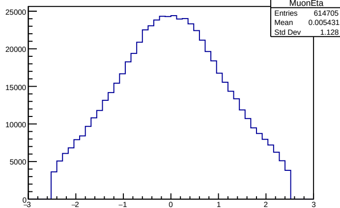
MuonEta
