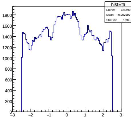
histEta
