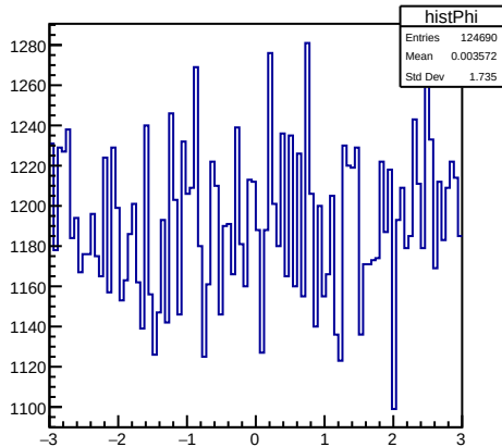
histPhi
