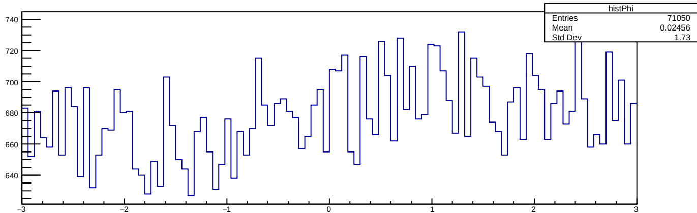
histPhi
