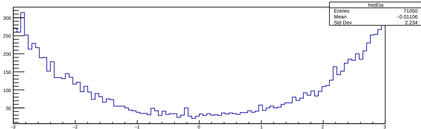
histEta
