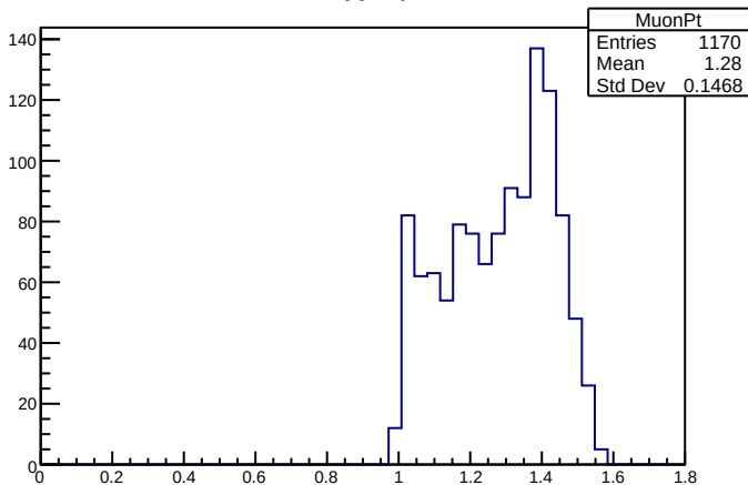
MuonPt
