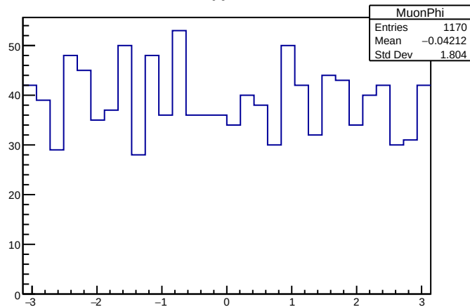
MuonPhi
