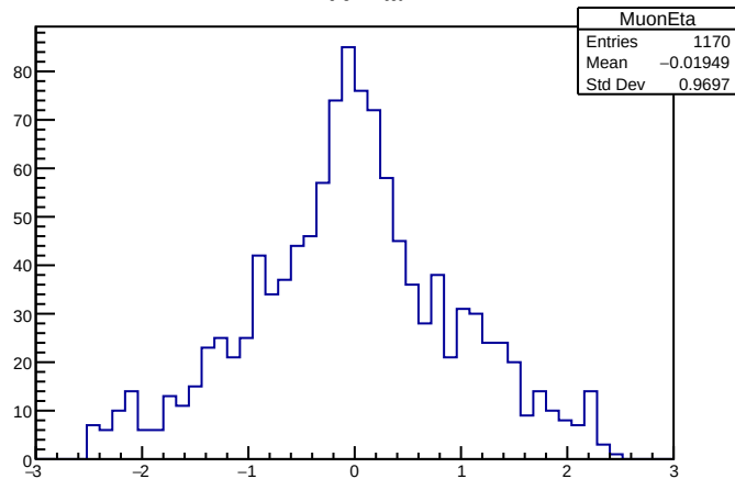
MuonEta
