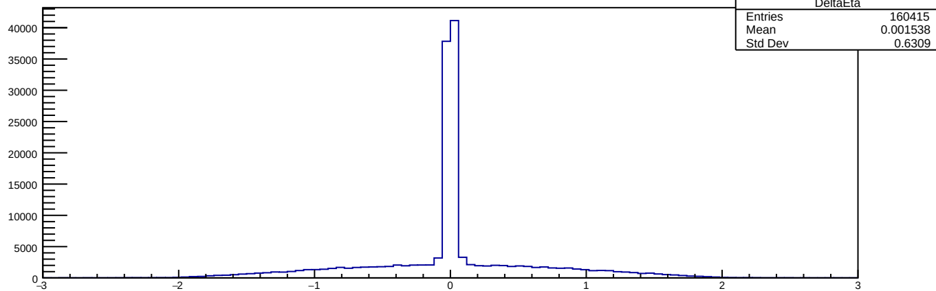
DeltaEta
