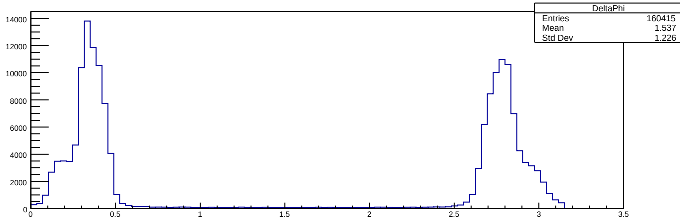
DeltaPhi
