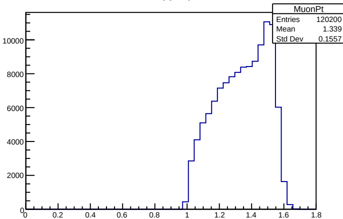
MuonPt
