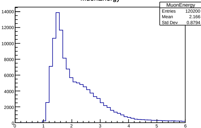
MuonEnergy
