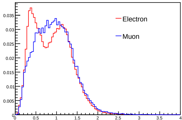
FMuon
