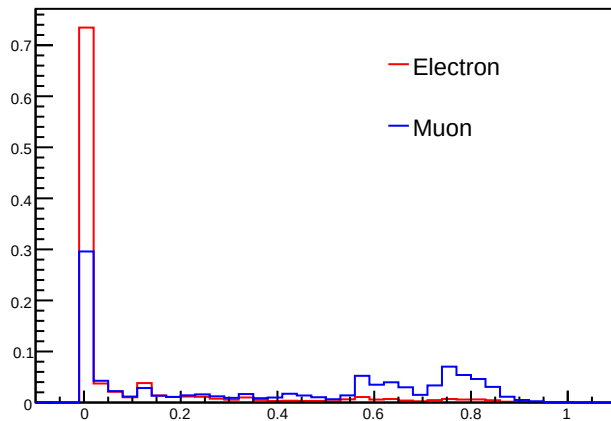
EMMuon
