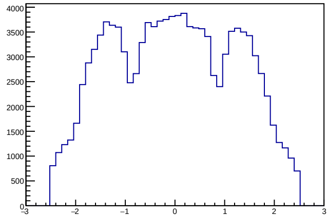
MuonEta
