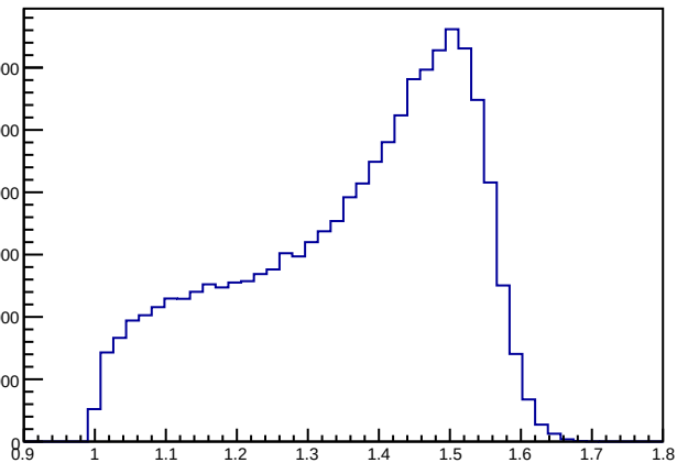
MuonPt
