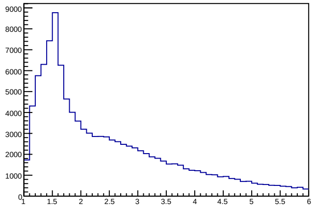
MuonEnergy
