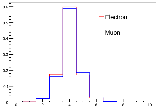
PixelEdX
