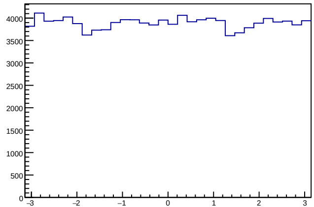
MuonPhi
