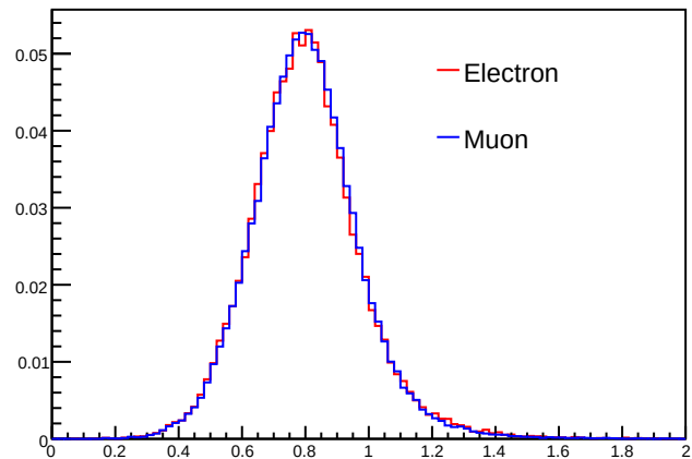
PixelEdX
