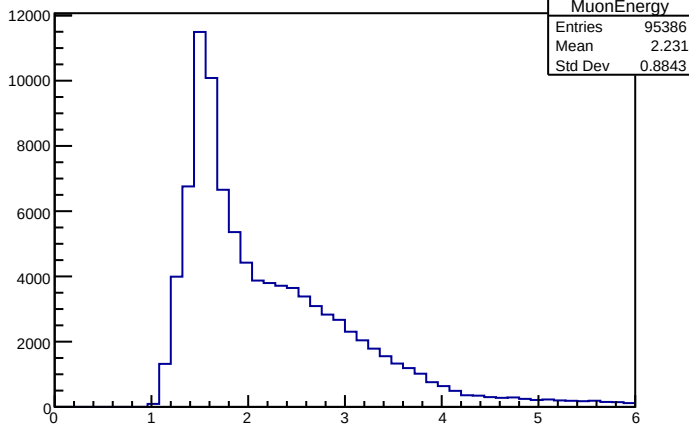
MuonEnergy
