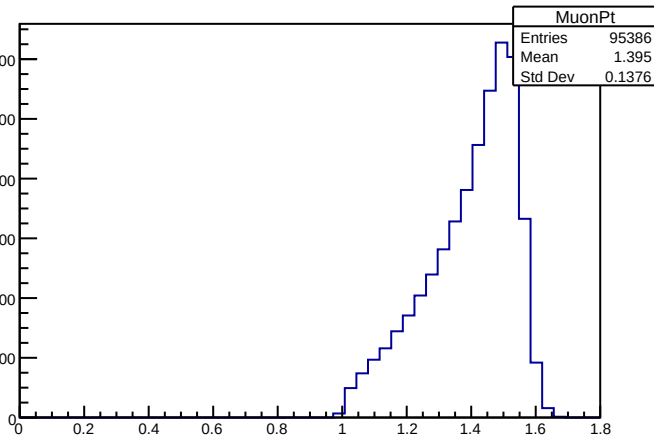
MuonPt
