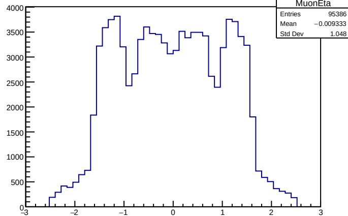
MuonEta
