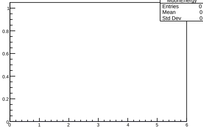
MuonEnergy
